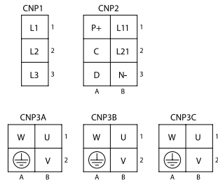
Anordnung der Steckverbindungen
