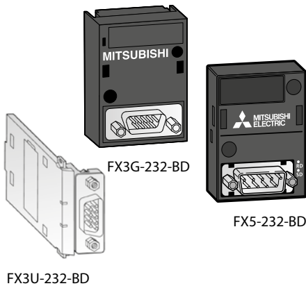
FX3U-232-BD
