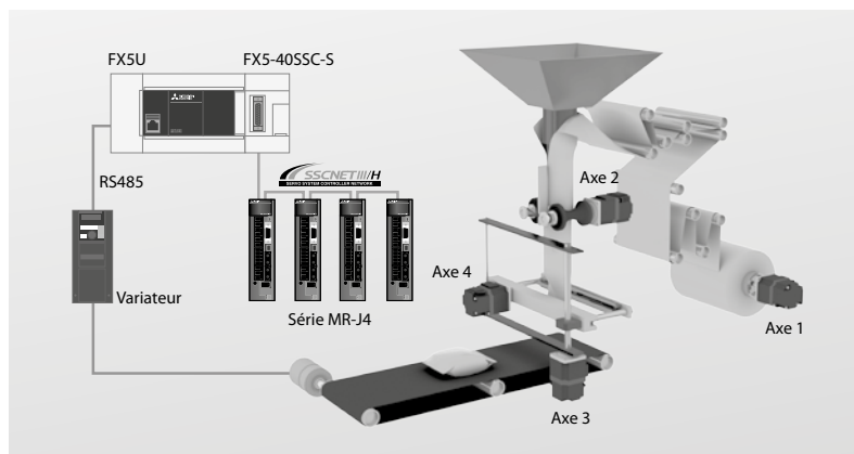
Machine d'emballage avec Simple Motion
