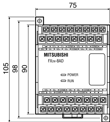
FX2N-8AD
