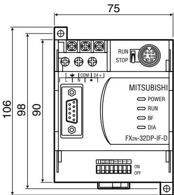
FX2N-32DP-IF-D
