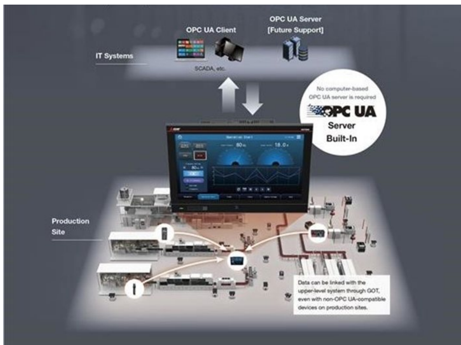
Bild 2: Mit dem integrierten OPC-UA-Server dient der GOT3000 als Gateway und ermöglicht die Datenintegration zwischen IT- und OT-Systemen.
