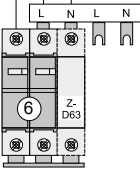
TN-S-/TT-System 1 x 230 VAC (1 x 220 VAC) (1 x 240 VAC)
