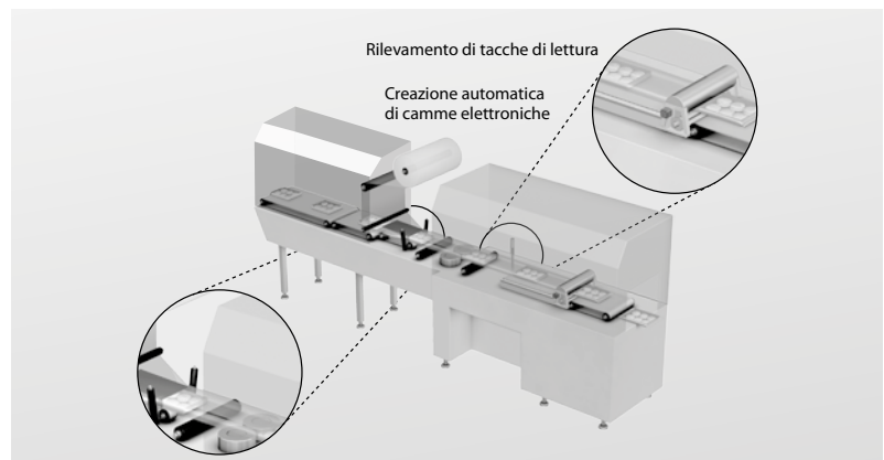
Taglierina a lama rotante con rilevamento tacche di lettura e dati della camma elettronica
