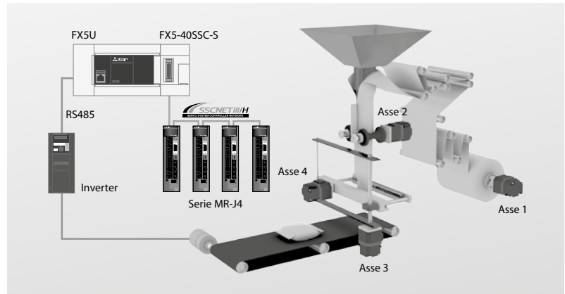
Macchina confezionatrice con Simple Motion
