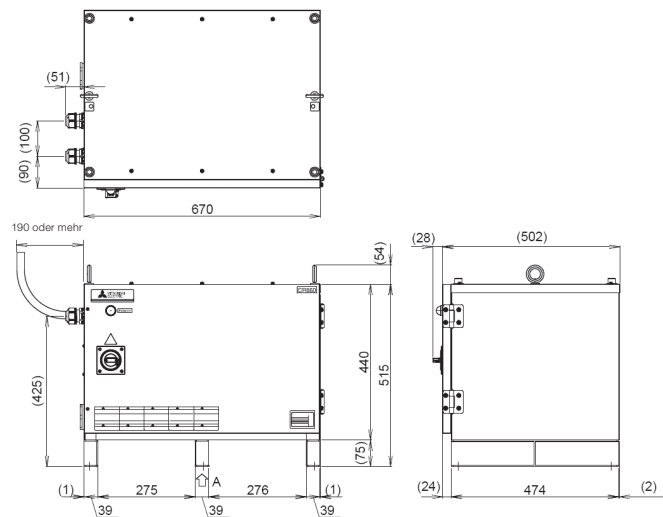
Transformatoreinheit CR860
