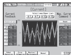
Menü zur Anzeige des Stroms und Lastfaktors
