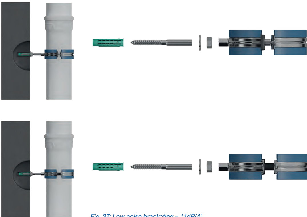
Fig. 37: Low noise bracketing – 14dB(A).
