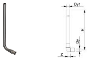
Tigris M5 radiatortilslutningsrør
