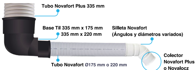
Conexión al elevador con tubería Novafort
