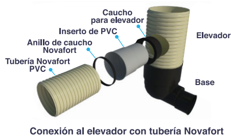
Conexión al elevador con tubería Novafort
