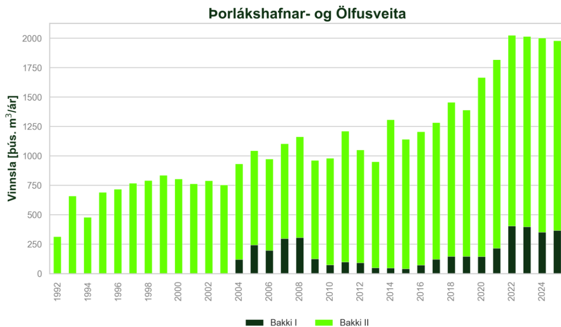
Mynd 2: Árleg heildarvinnsla Þorlákshafnar- og Ölfusveitu árin 1992-2025.
