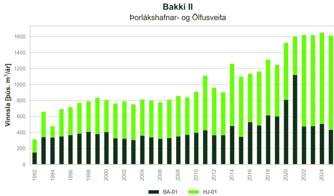
Mynd 4: Árleg vinnsla úr holum á Bakka II árin 1992-2025.
