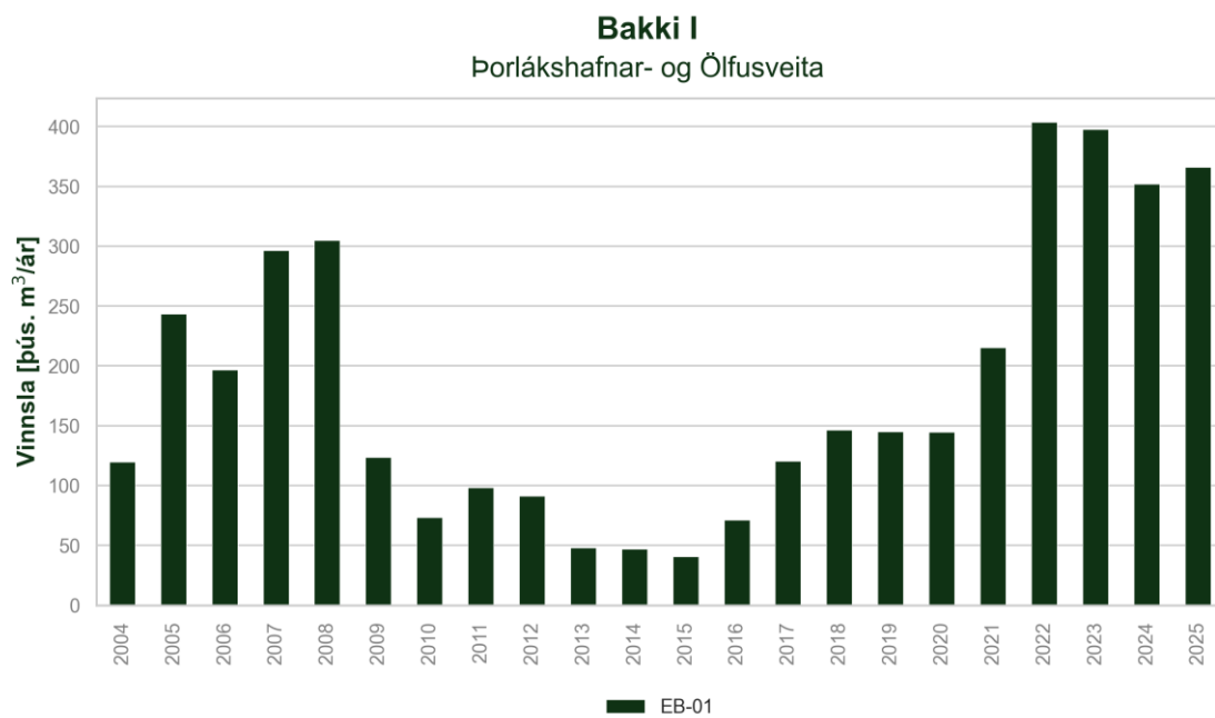
Mynd 3: Árleg vinnsla úr holum á Bakka I árin 2004-2025.
