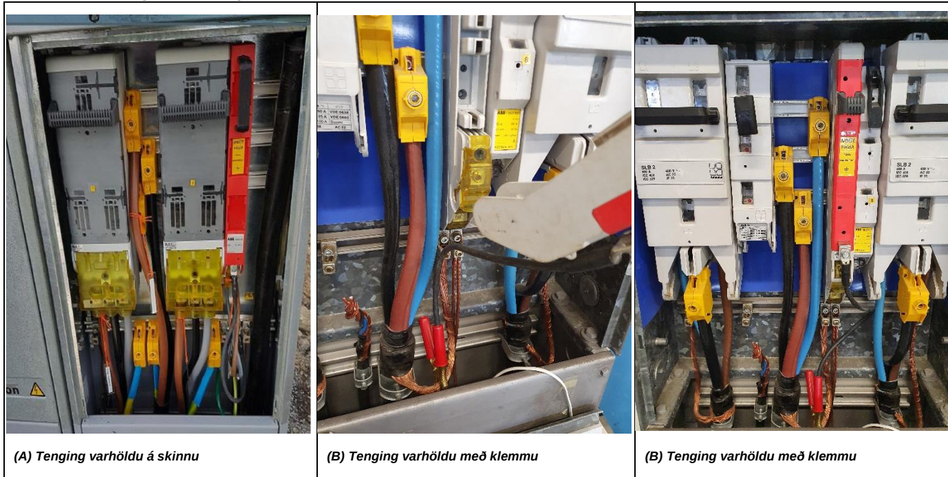
Mynd 1: Útfærslur A og B í götuvarskáp
