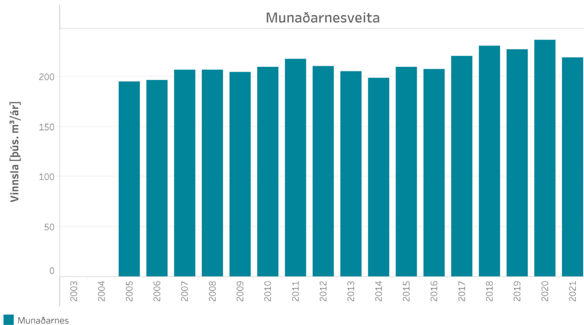
Mynd 2. Árleg heildarvinnsla Munaðarnesveitu árin 2005-2021.
