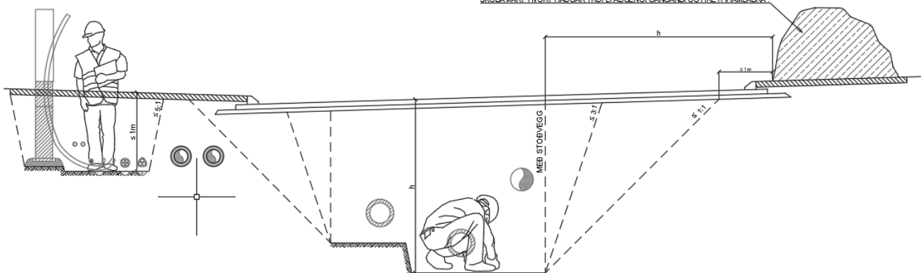
Mynd 14: Öryggi við skurðgröft og gryfjur (LAV-131)
