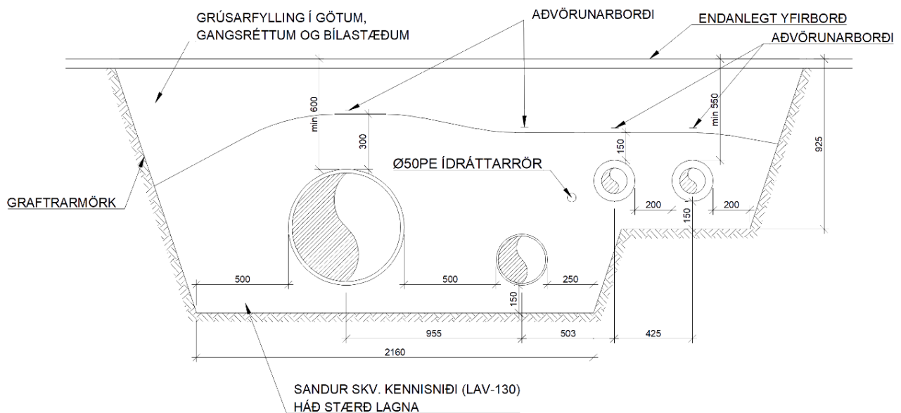
Mynd 27: Málsetningar með skálinum.
