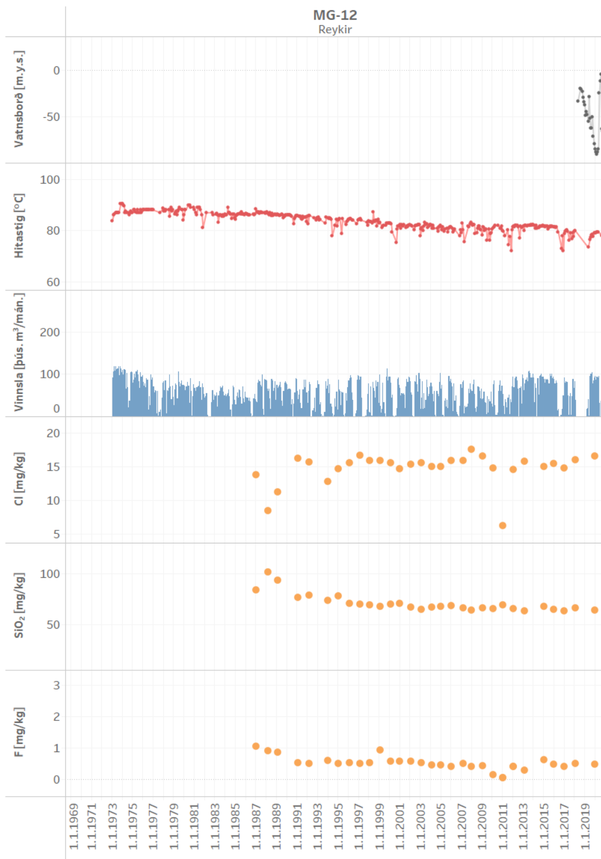
Mynd 34. Vinnsla úr holu MG-12 ásamt breytingum á vatnsborði, hita og efnainnihaldi
