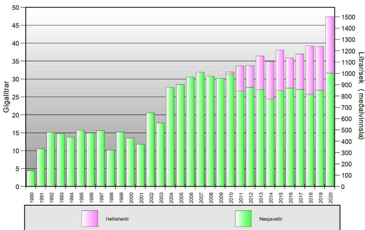
Mynd 64. Nesjavellir og Hellisheiði. Árleg vinnsla 1990 - 2020
