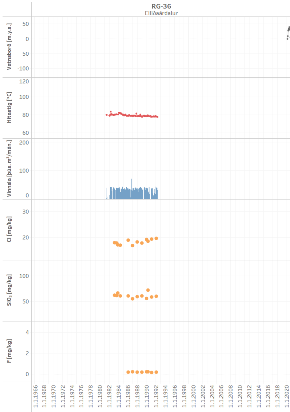
Mynd 23. Vinnsla úr holu RG-36 ásamt breytingum á vatnsborði, hita og efnainnihaldi
