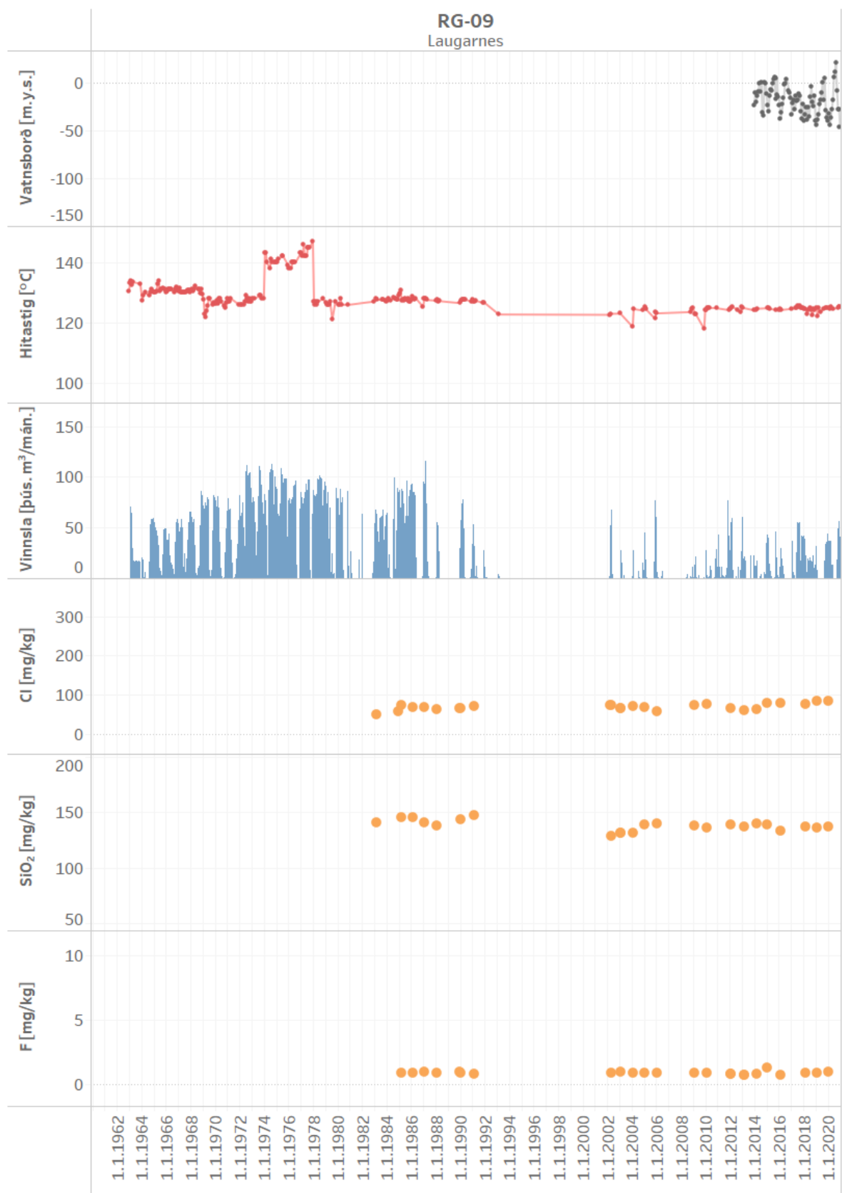
Mynd 7. Vinnsla úr holu RG-09 ásamt breytingum á vatnsborði, hita og efnainnihaldi
