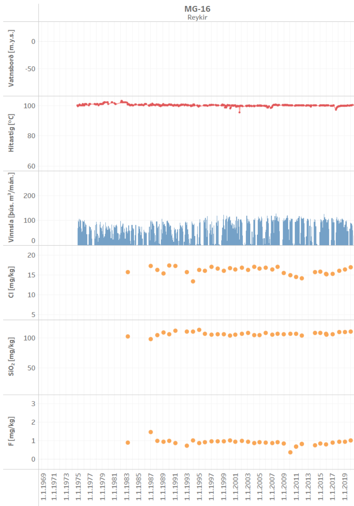
Mynd 38. Vinnsla úr holu MG-16 ásamt breytingum á vatnsborði, hita og efnainnihaldi
