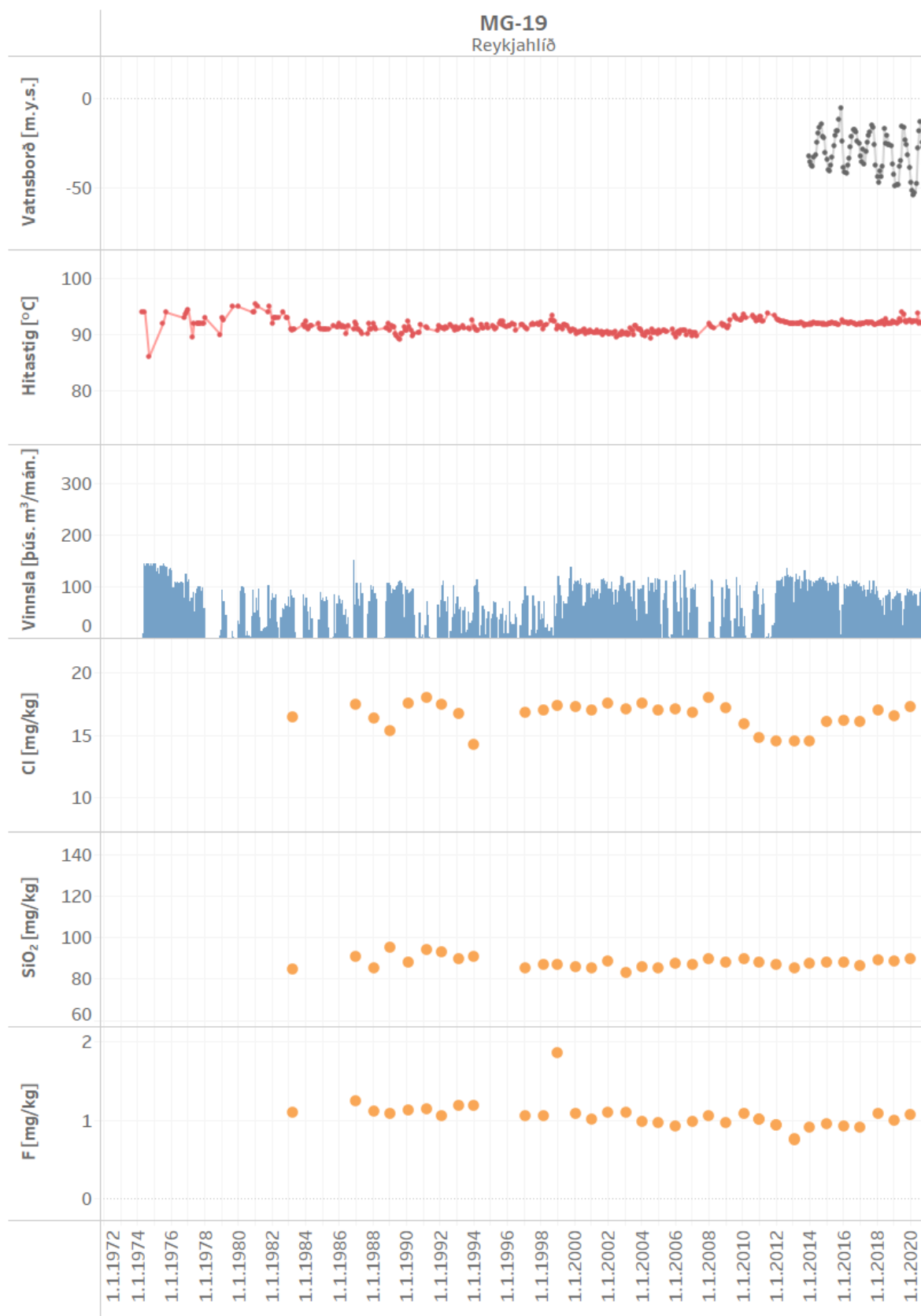
Mynd 53. Vinnsla úr holu MG-19 ásamt breytingum á vatnsborði, hita og efnainnihaldi
