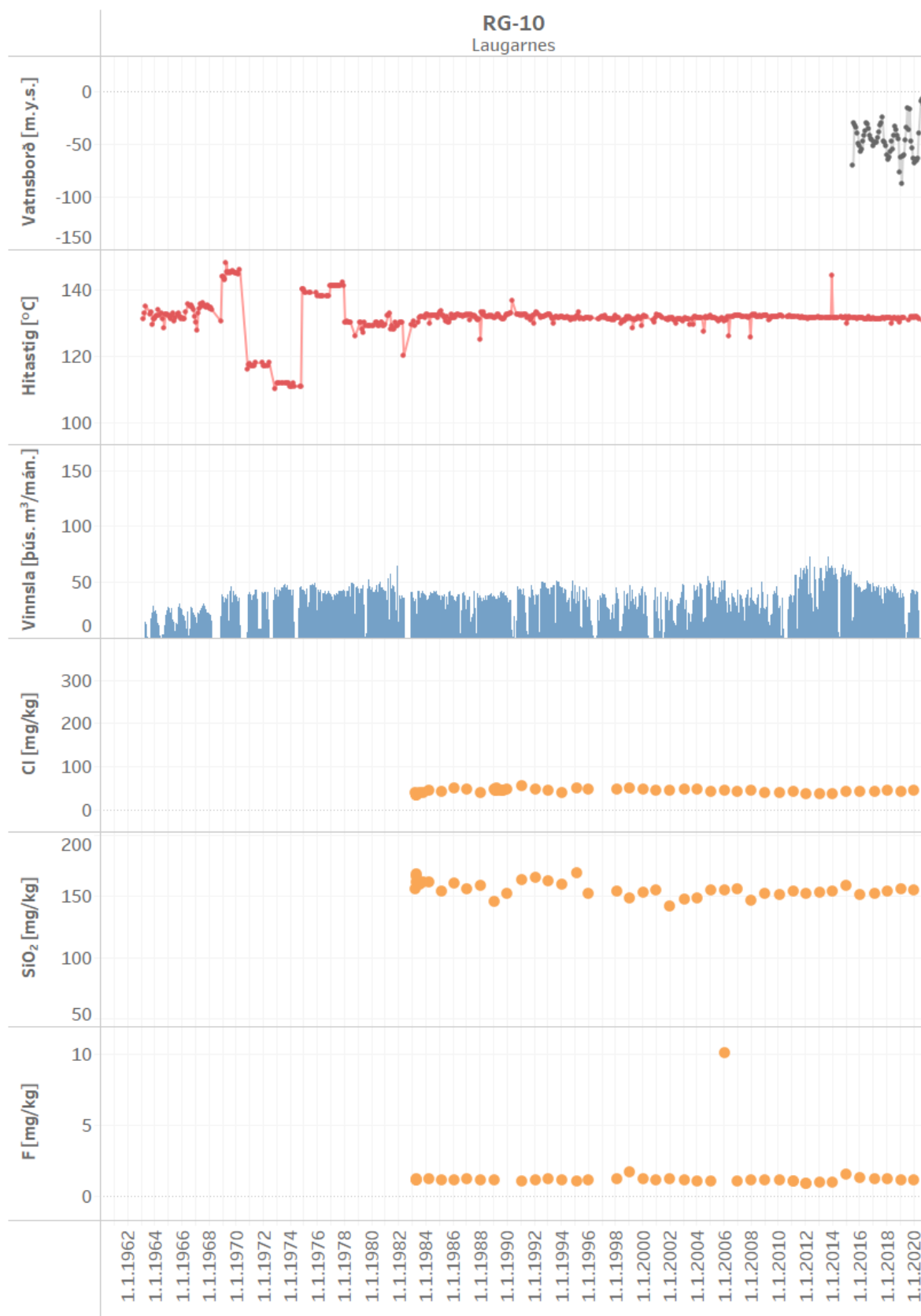
Mynd 8. Vinnsla úr holu RG-10 ásamt breytingum á vatnsborði, hita og efnainnihaldi
