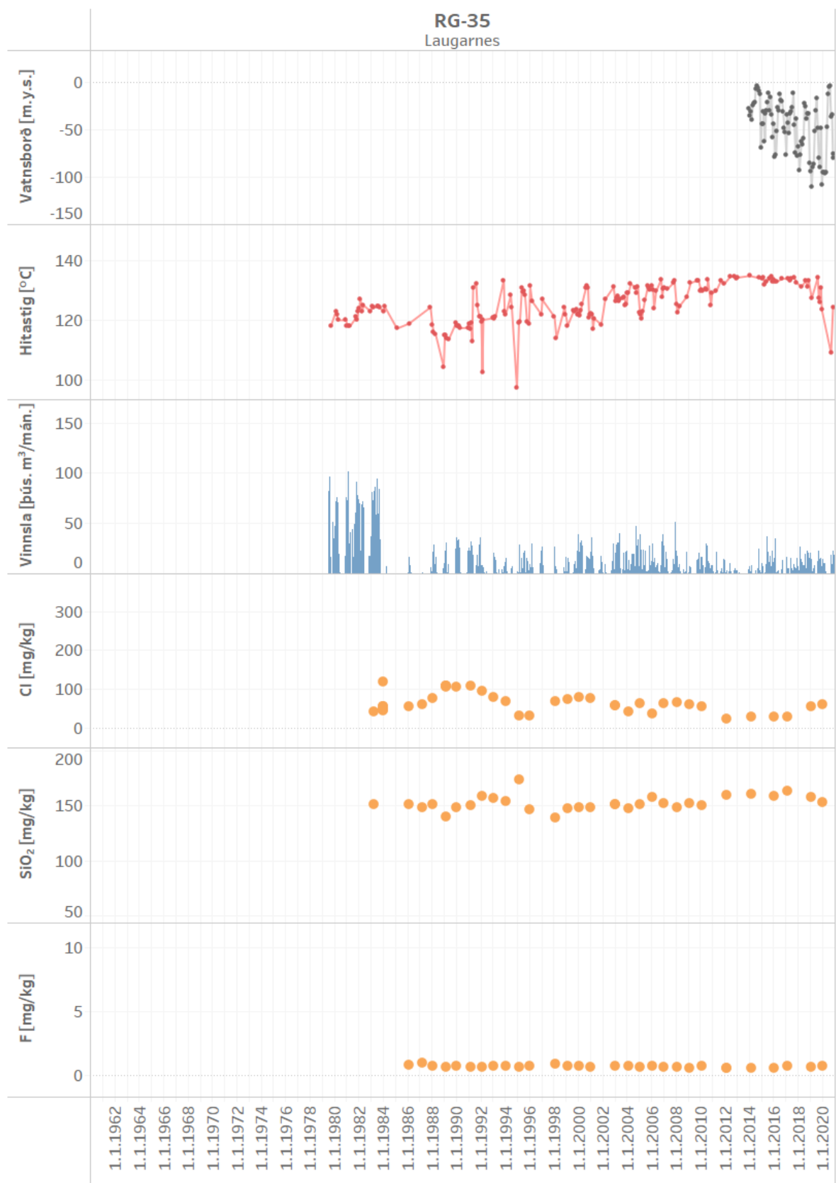
Mynd 14. Vinnsla úr holu RG-35 ásamt breytingum á vatnsborði, hita og efnainnihaldi
