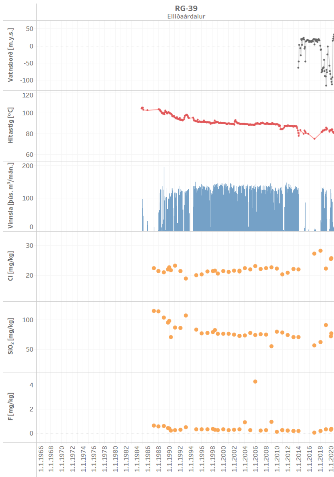
Mynd 25. Vinnsla úr holu RG-39 ásamt breytingum á vatnsborði, hita og efnainnihaldi
