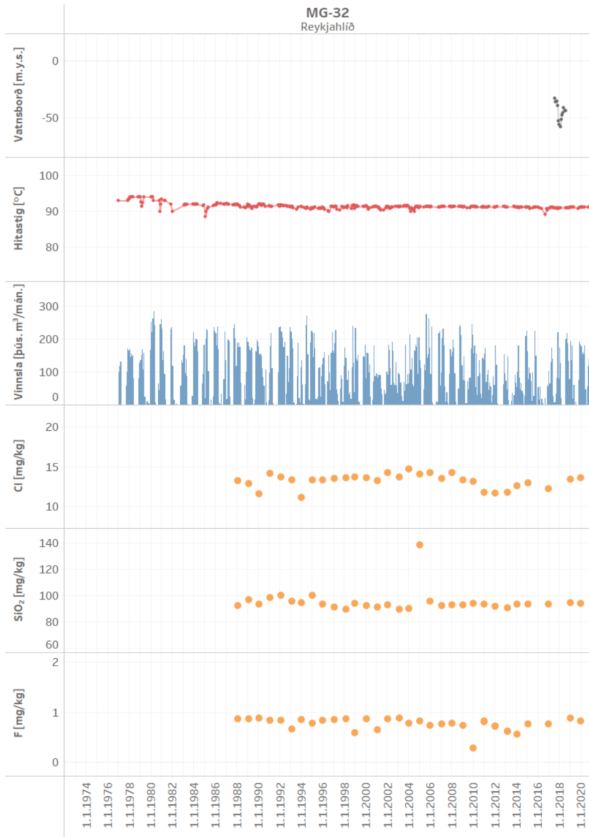
Mynd 56. Vinnsla úr holu MG-32 ásamt breytingum á vatnsborði, hita og efnainnihaldi
