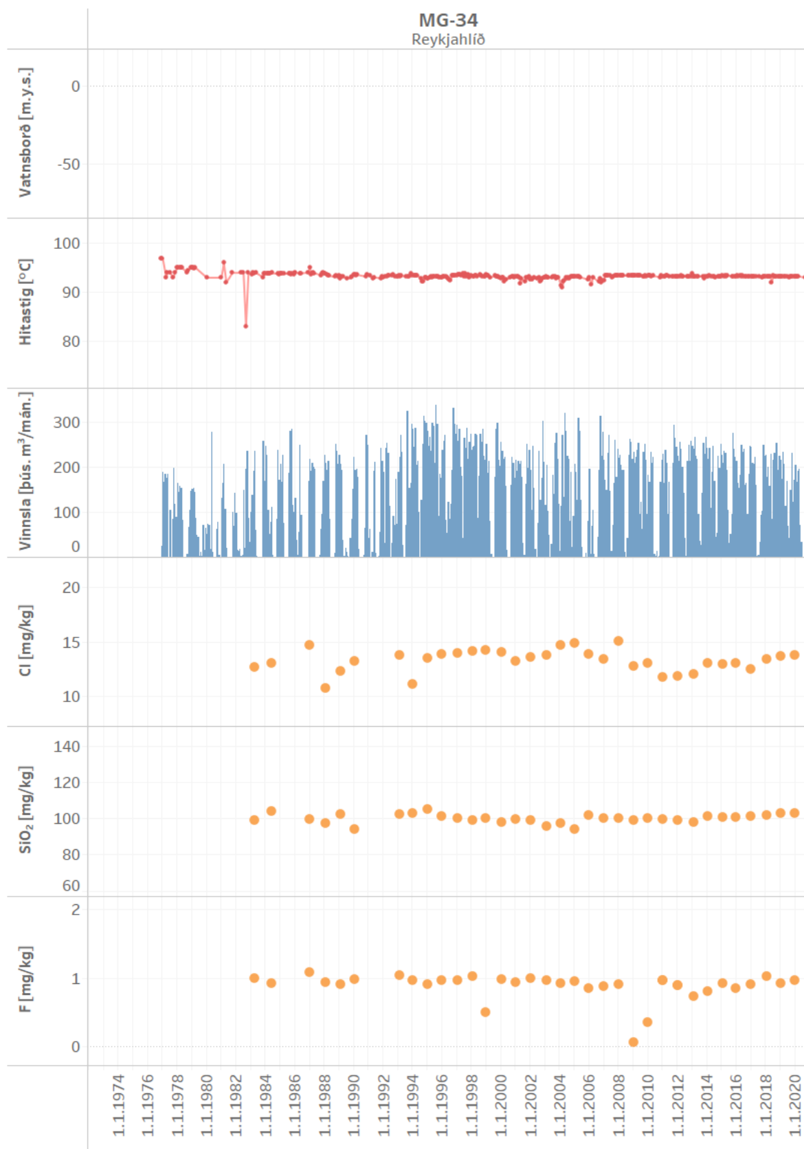
Mynd 58. Vinnsla úr holu MG-34 ásamt breytingum á vatnsborði, hita og efnainnihaldi
