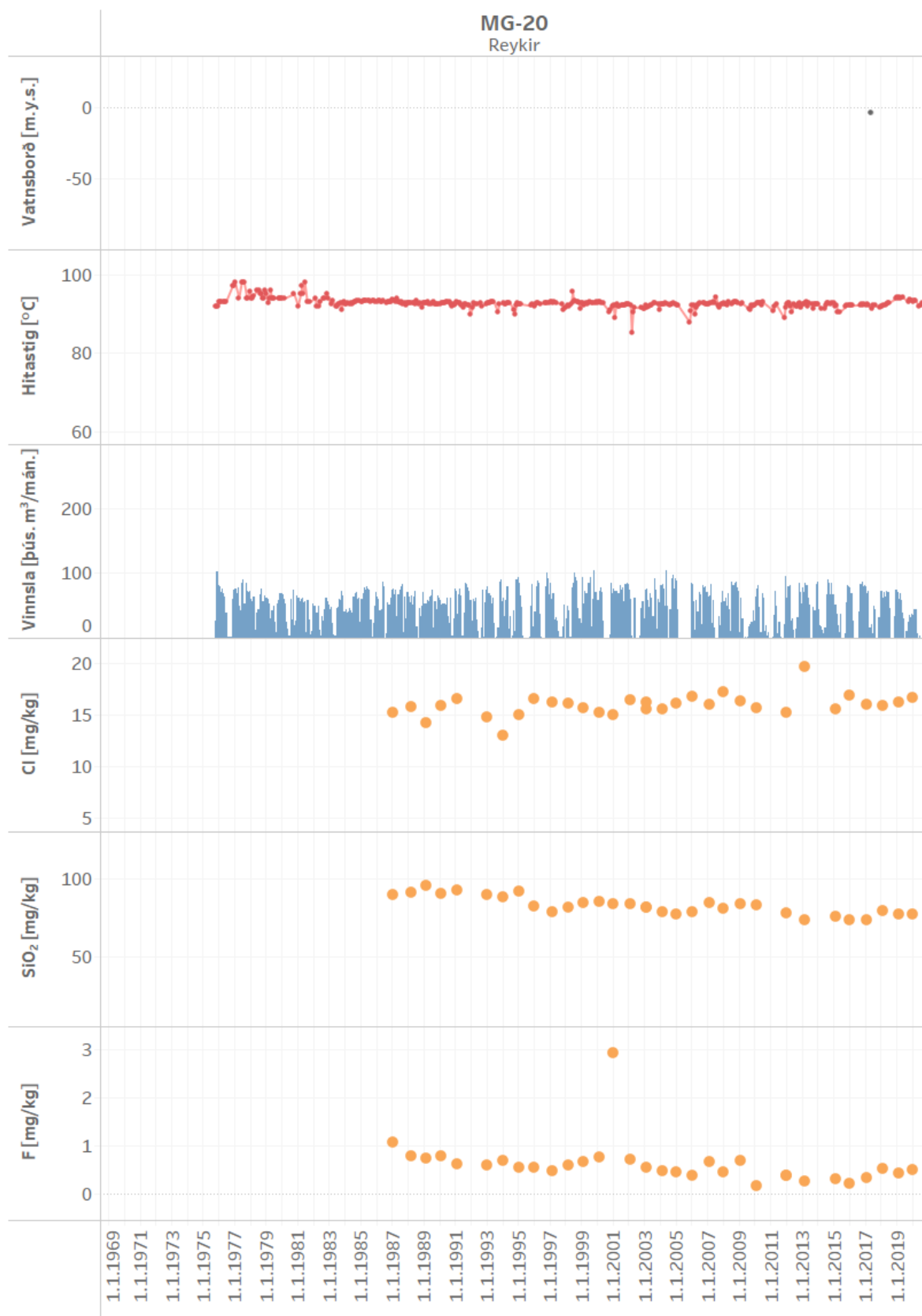
Mynd 41. Vinnsla úr holu MG-20 ásamt breytingum á vatnsborði, hita og efnainnihaldi
