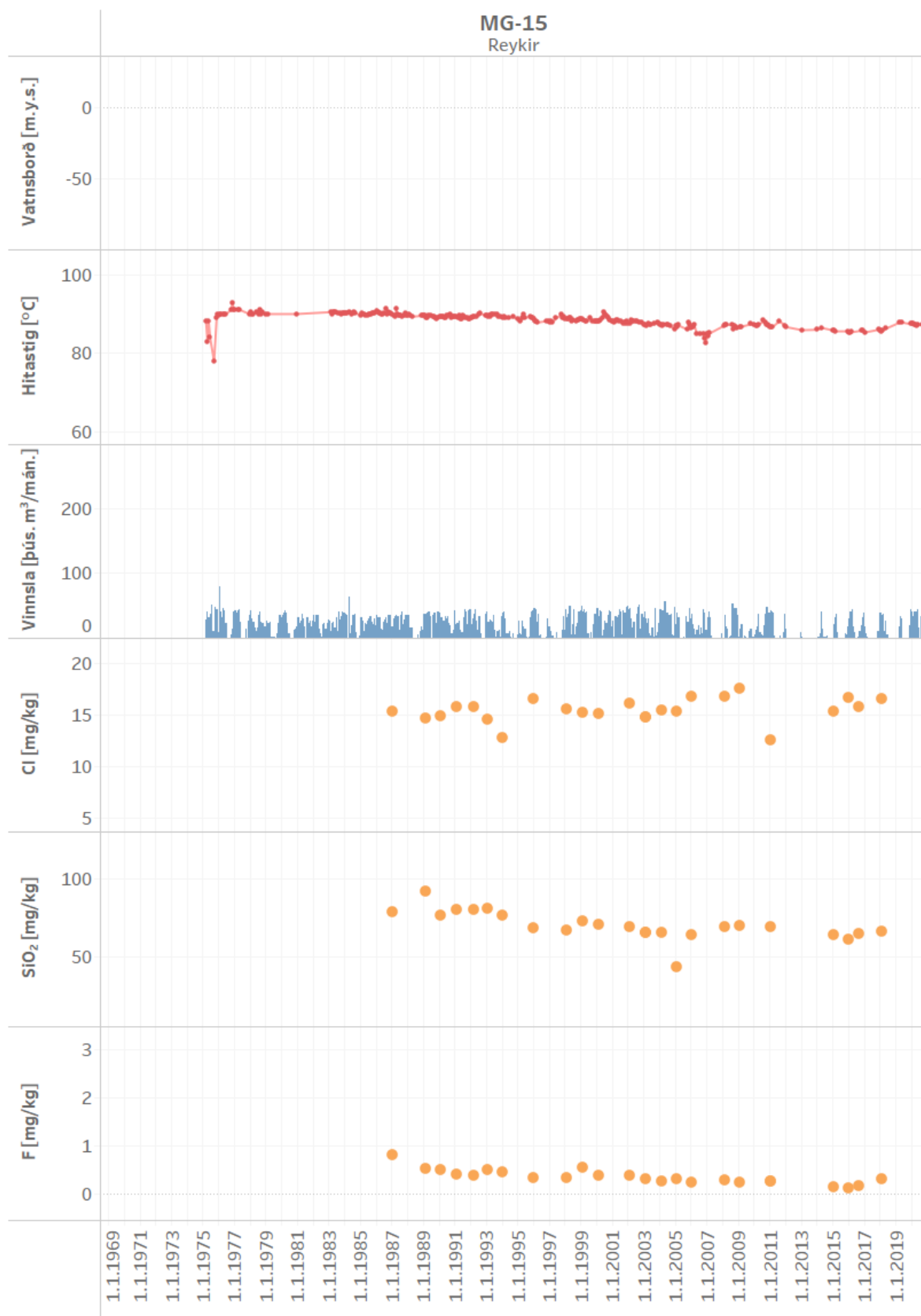
Mynd 37. Vinnsla úr holu MG-15 ásamt breytingum á vatnsborði, hita og efnainnihaldi
