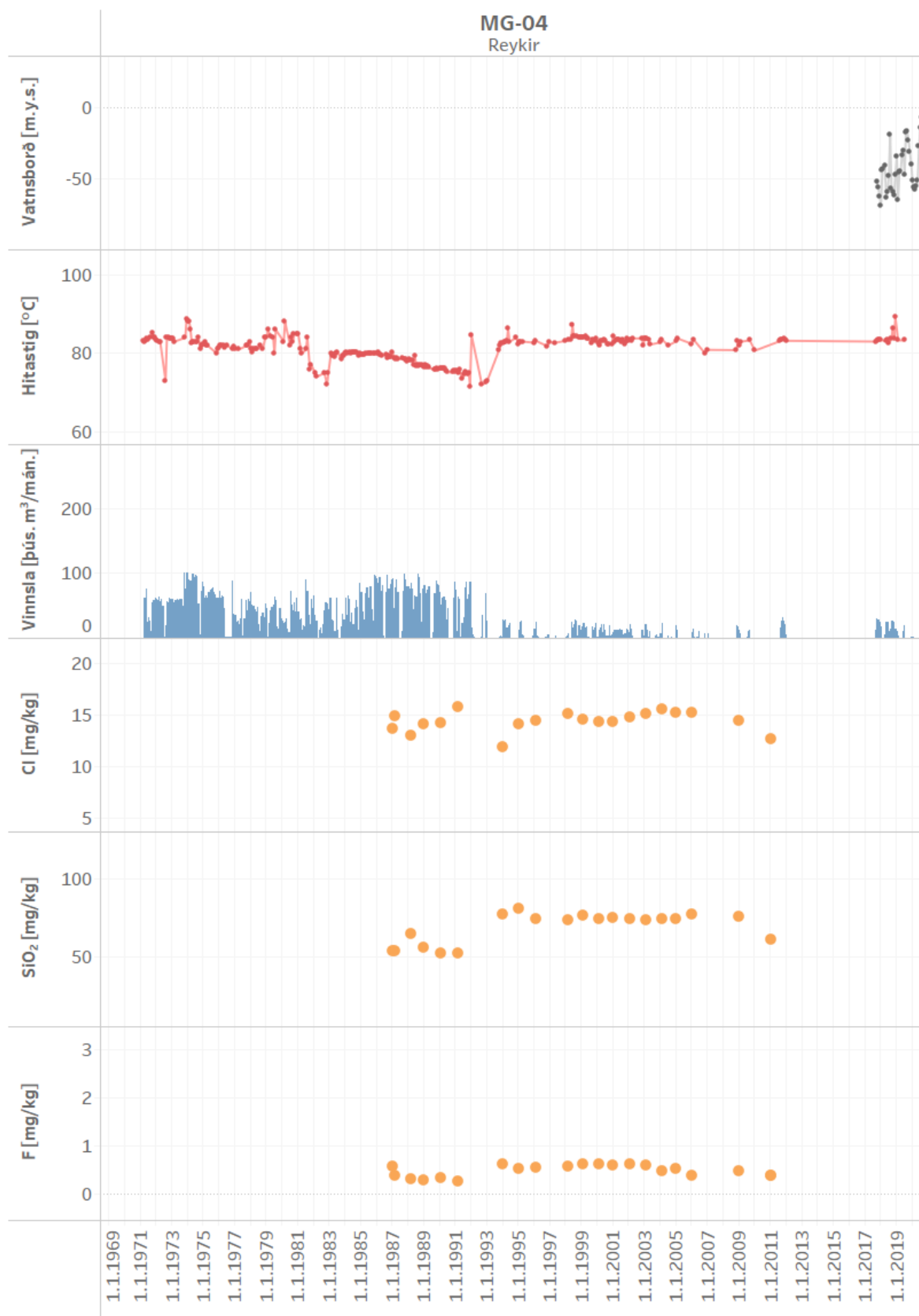
Mynd 29. Vinnsla úr holu MG-04 ásamt breytingum á vatnsborði, hita og efnainnihaldi
