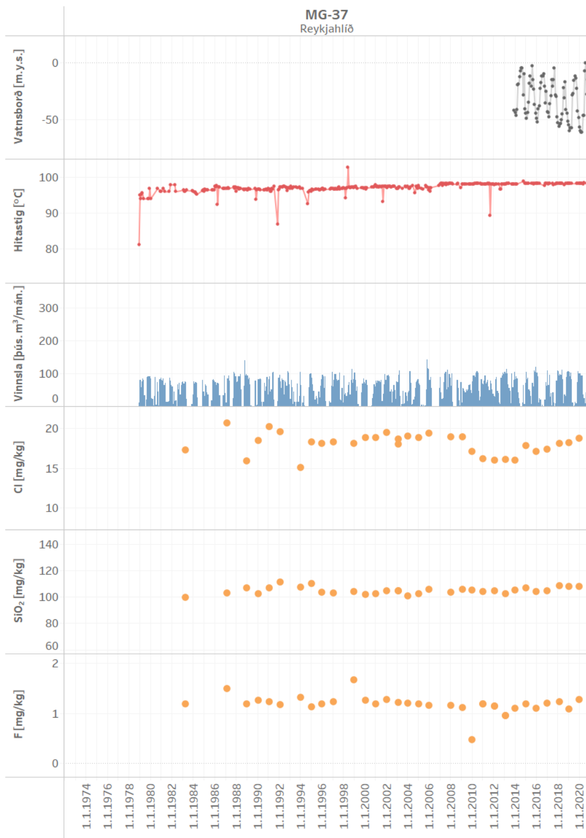
Mynd 61. Vinnsla úr holu MG-37 ásamt breytingum á vatnsborði, hita og efnainnihaldi
