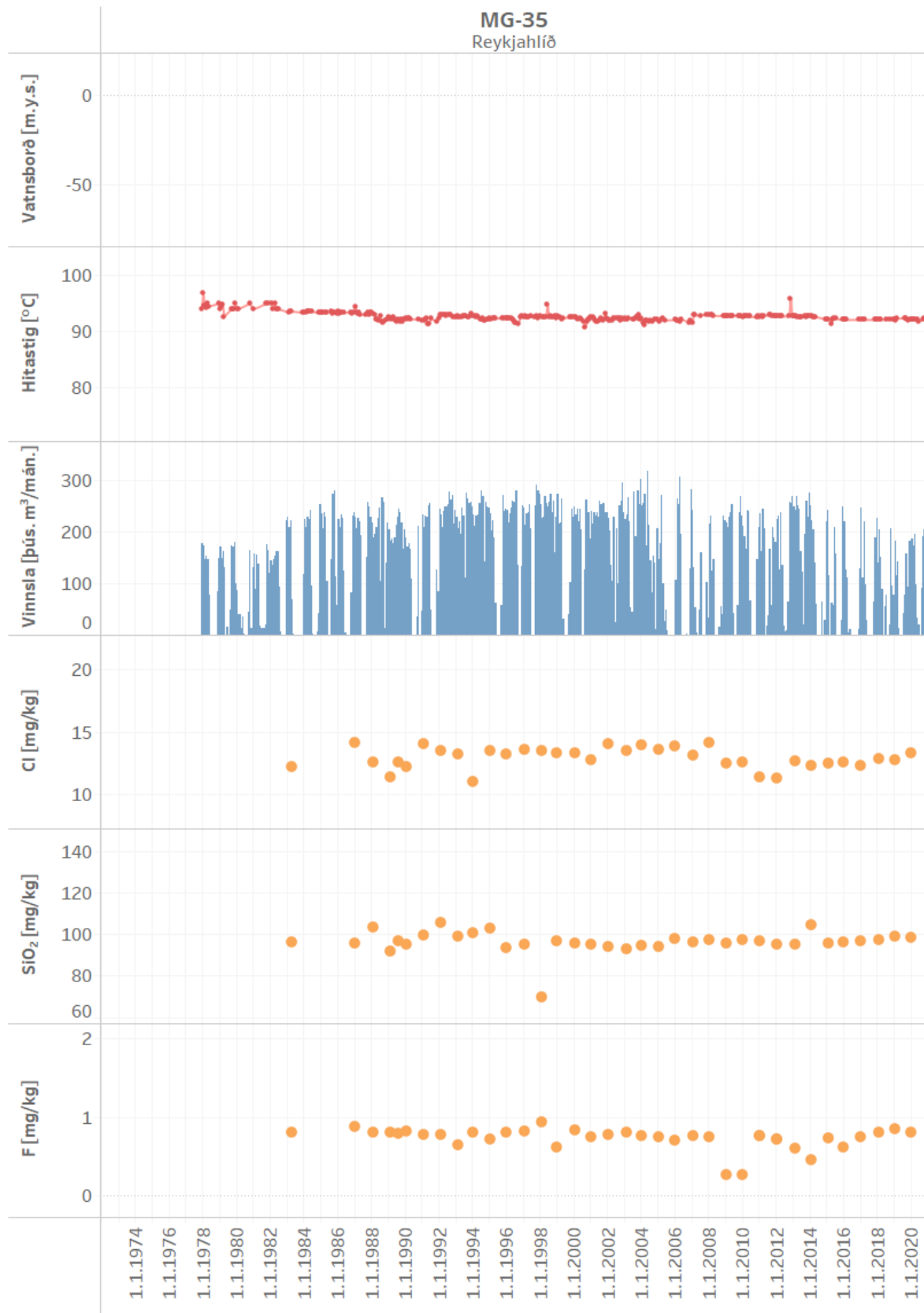
Mynd 59. Vinnsla úr holu MG-35 ásamt breytingum á vatnsborði, hita og efnainnihaldi
