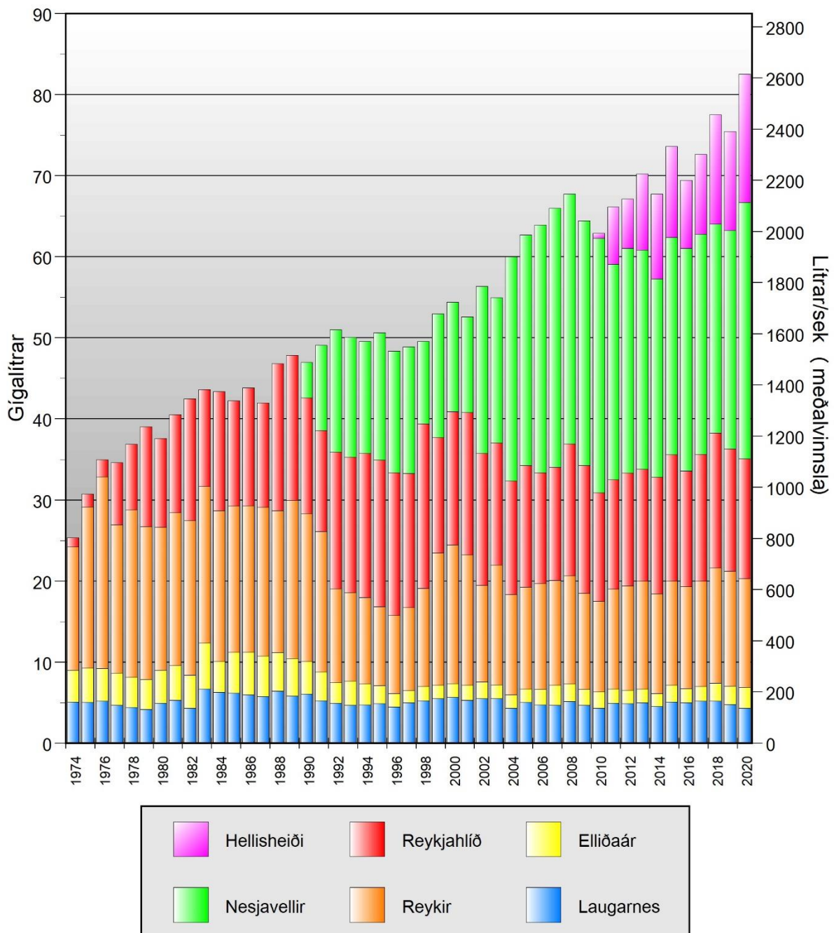
Mynd 2. Hitaveitunotkun á árunum 1974 – 2020 skipt eftir virkjunarsvæðum
