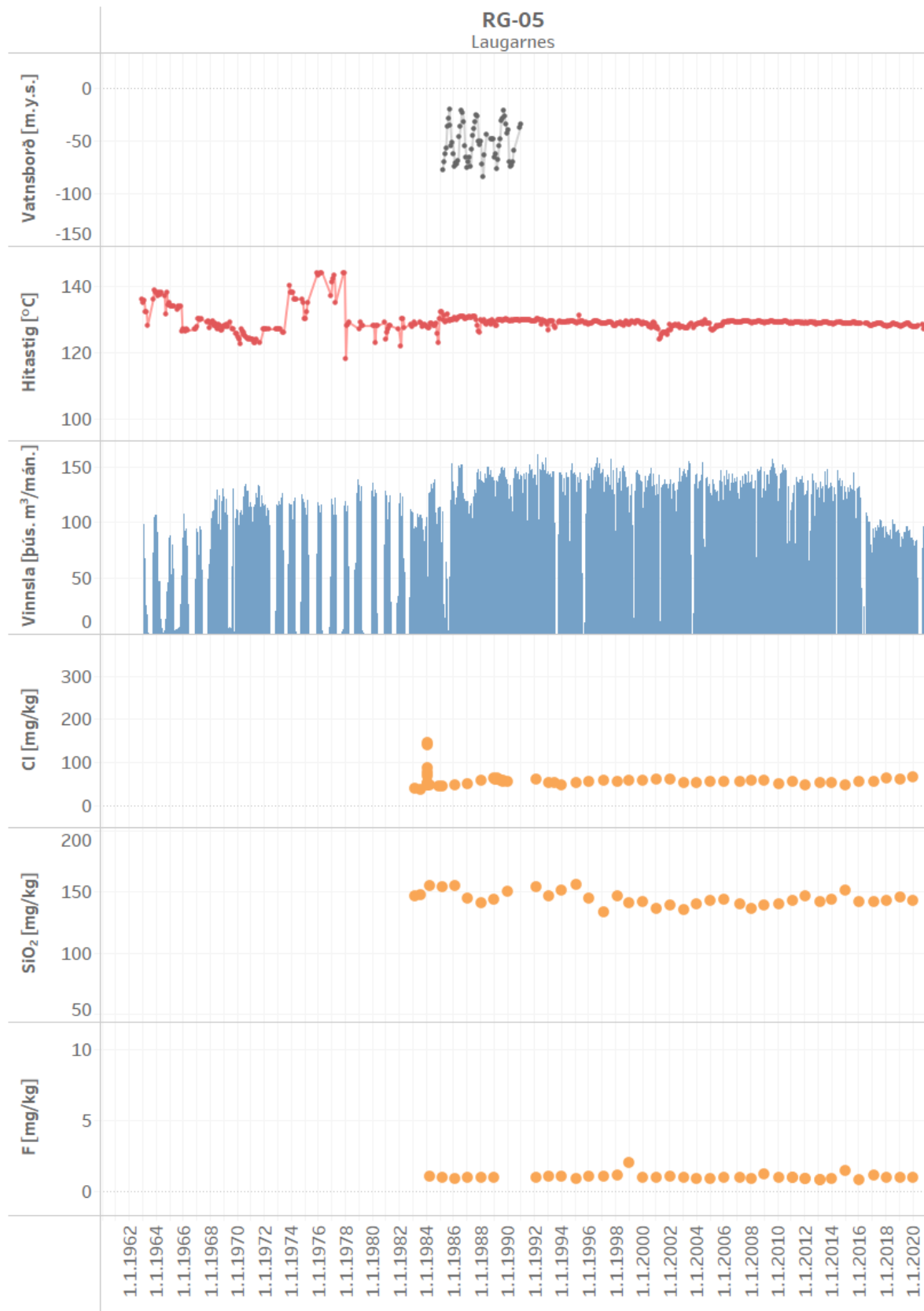
Mynd 6. Vinnsla úr holu RG-05 ásamt breytingum á vatnsborði, hita og efnainnihaldi
