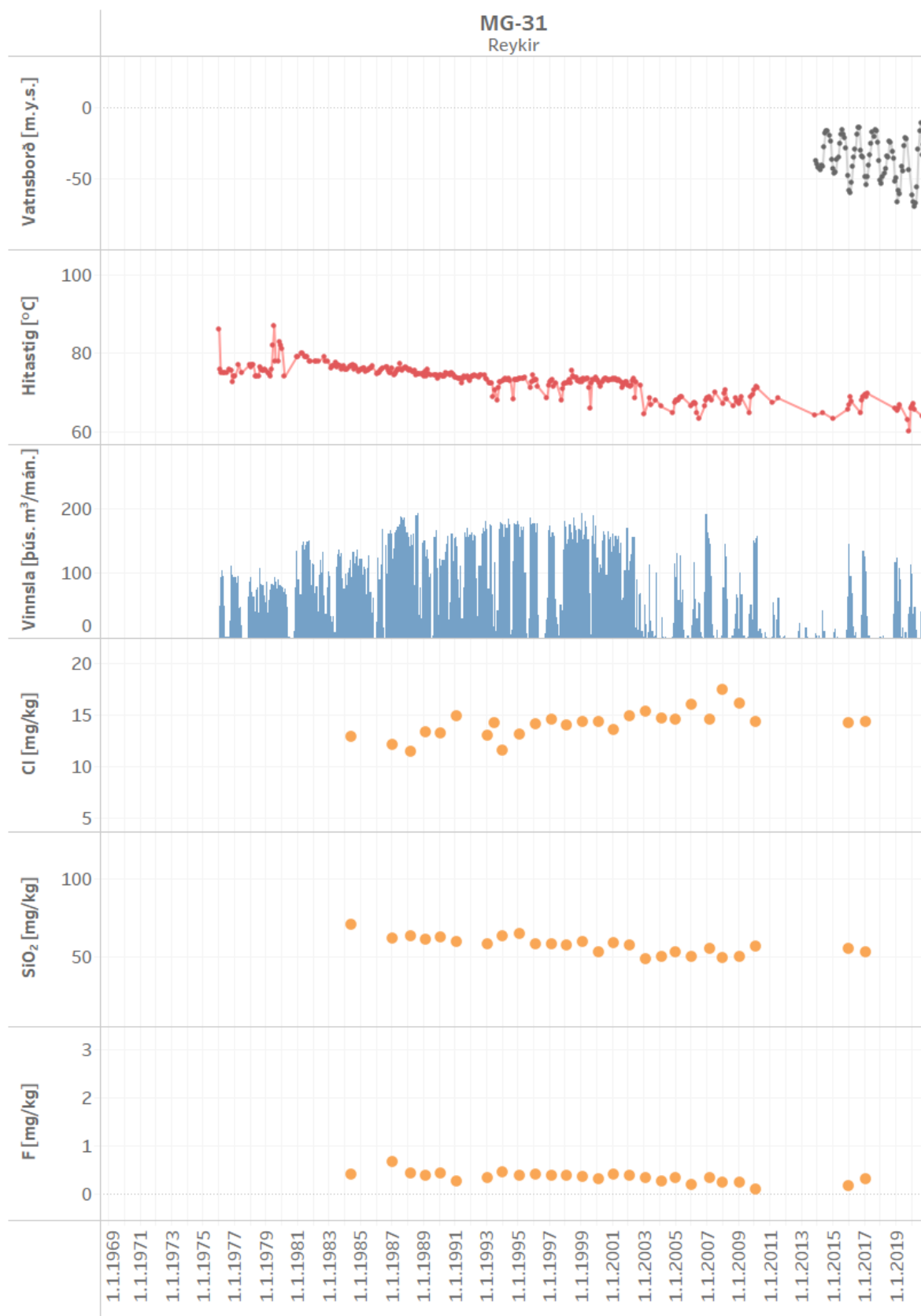
Mynd 49. Vinnsla úr holu MG-31 ásamt breytingum á vatnsborði, hita og efnainnihaldi
