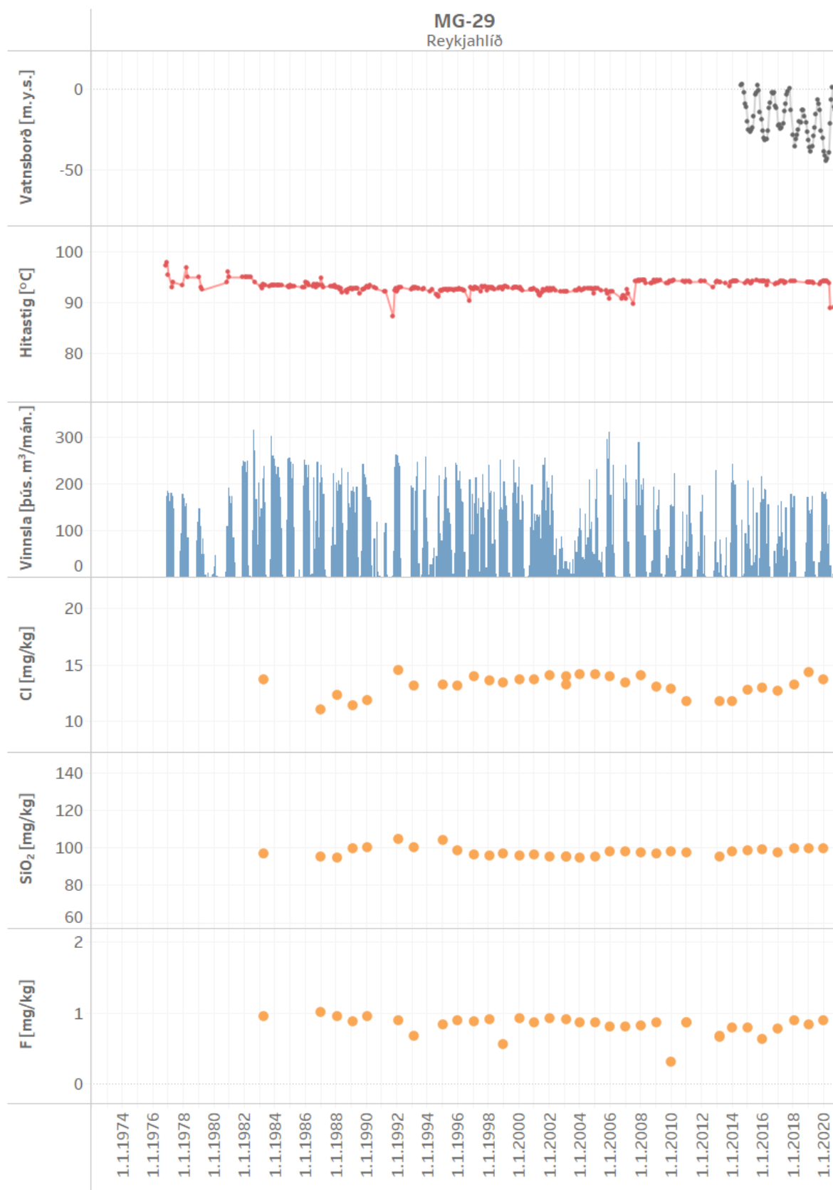
Mynd 55. Vinnsla úr holu MG-29 ásamt breytingum á vatnsborði, hita og efnainnihaldi
