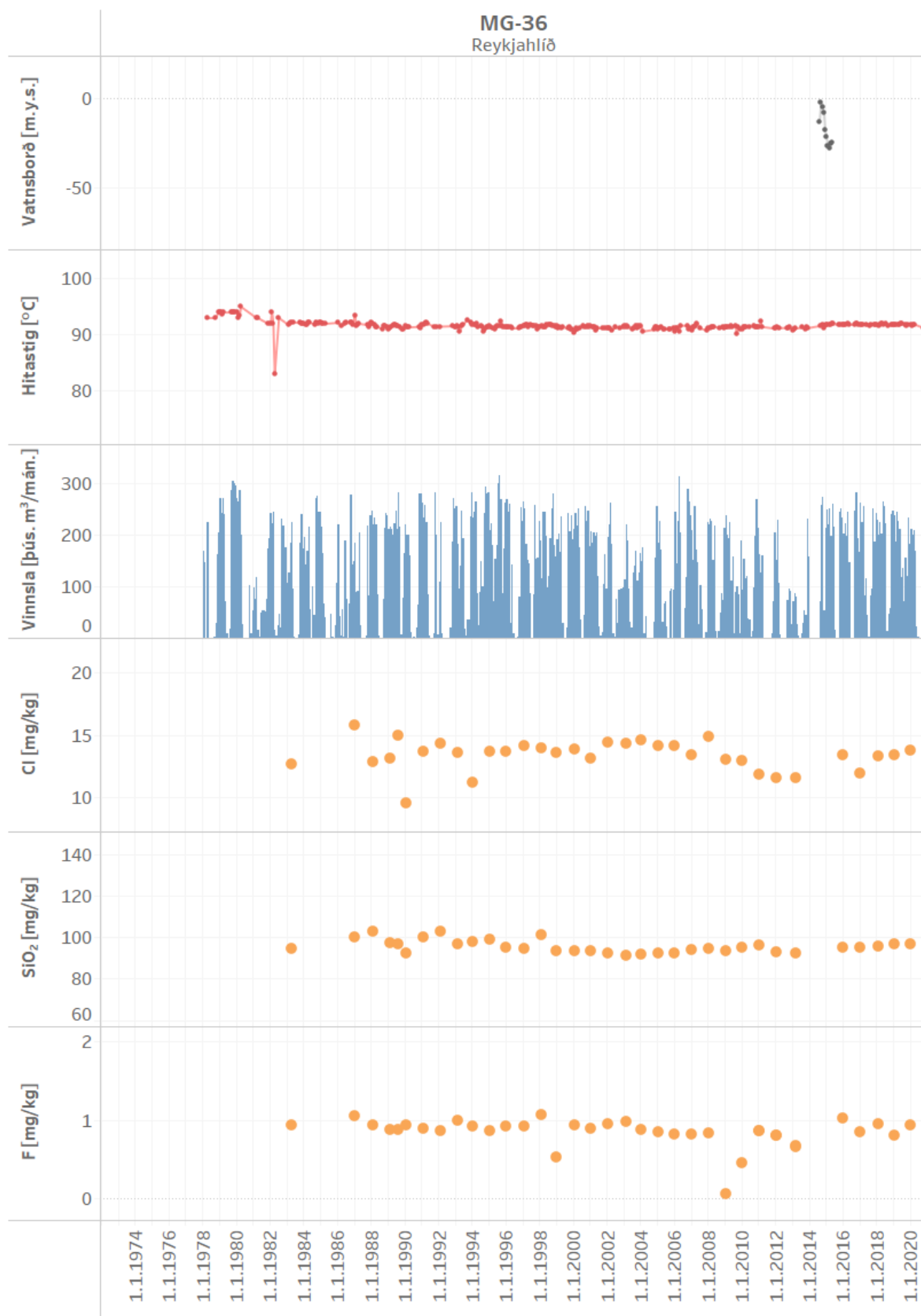
Mynd 60. Vinnsla úr holu MG-36 ásamt breytingum á vatnsborði, hita og efnainnihaldi
