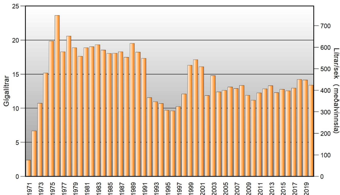
Mynd 26. Árleg heildarvinnsla Reykjasvæðisins árin 1971 - 2020
