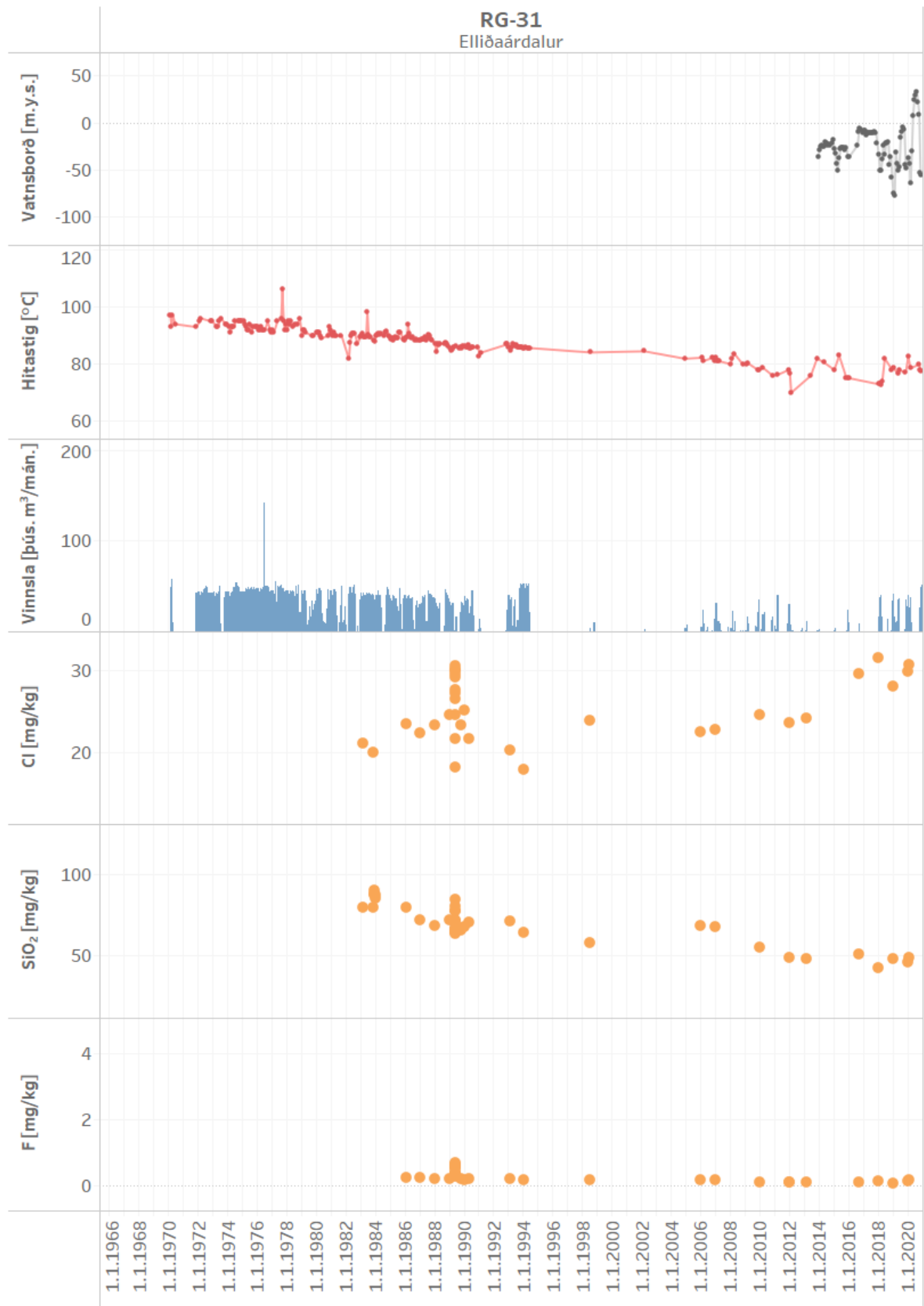
Mynd 22. Vinnsla úr holu RG-31 ásamt breytingum á vatnsborði, hita og efnainnihaldi
