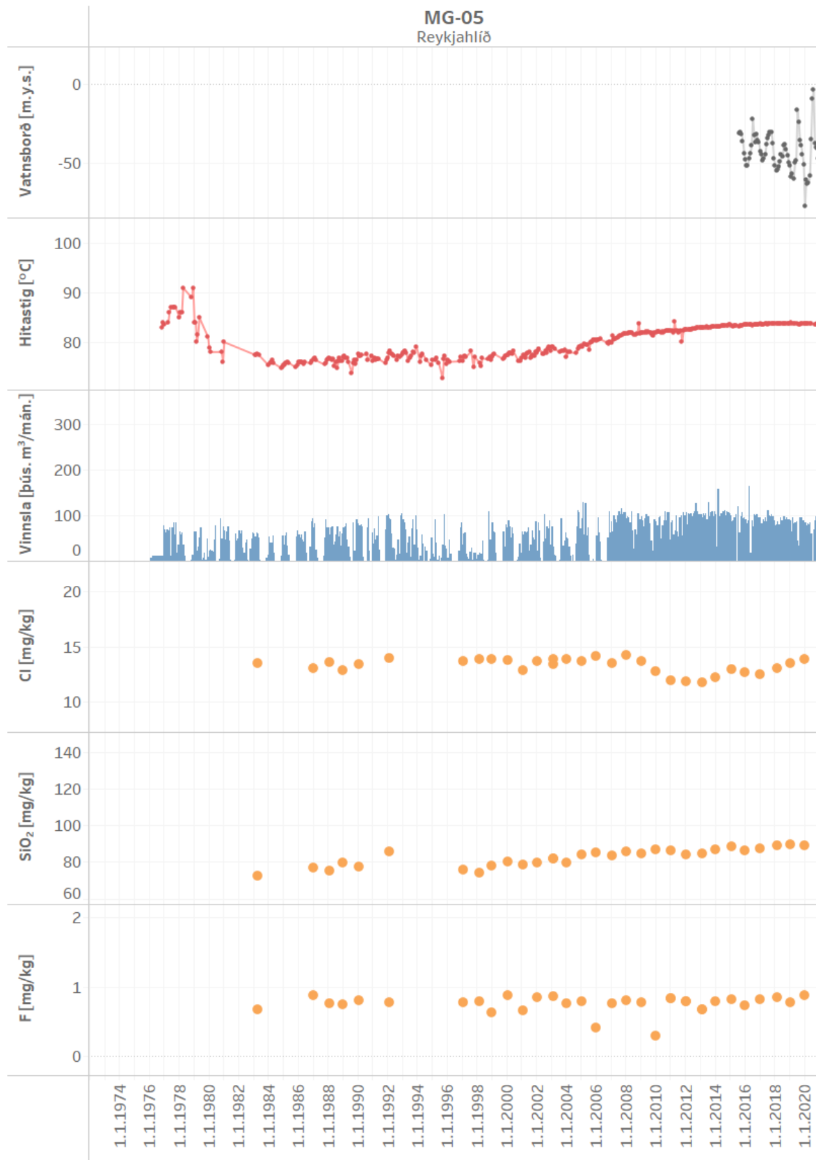
Mynd 52. Vinnsla úr holu MG-05 ásamt breytingum á vatnsborði, hita og efnainnihaldi
