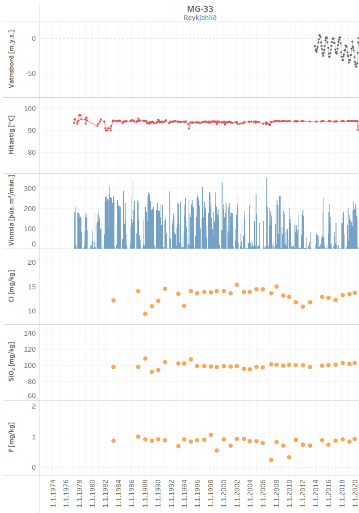
Mynd 57. Vinnsla úr holu MG-33 ásamt breytingum á vatnsborði, hita og efnainnihaldi
