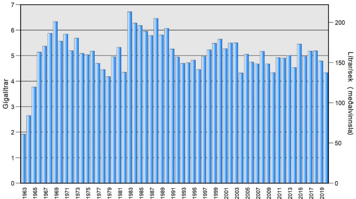
Mynd 4. Árleg heildarvinnsla Laugarnessvæðisins árin 1963 - 2020
