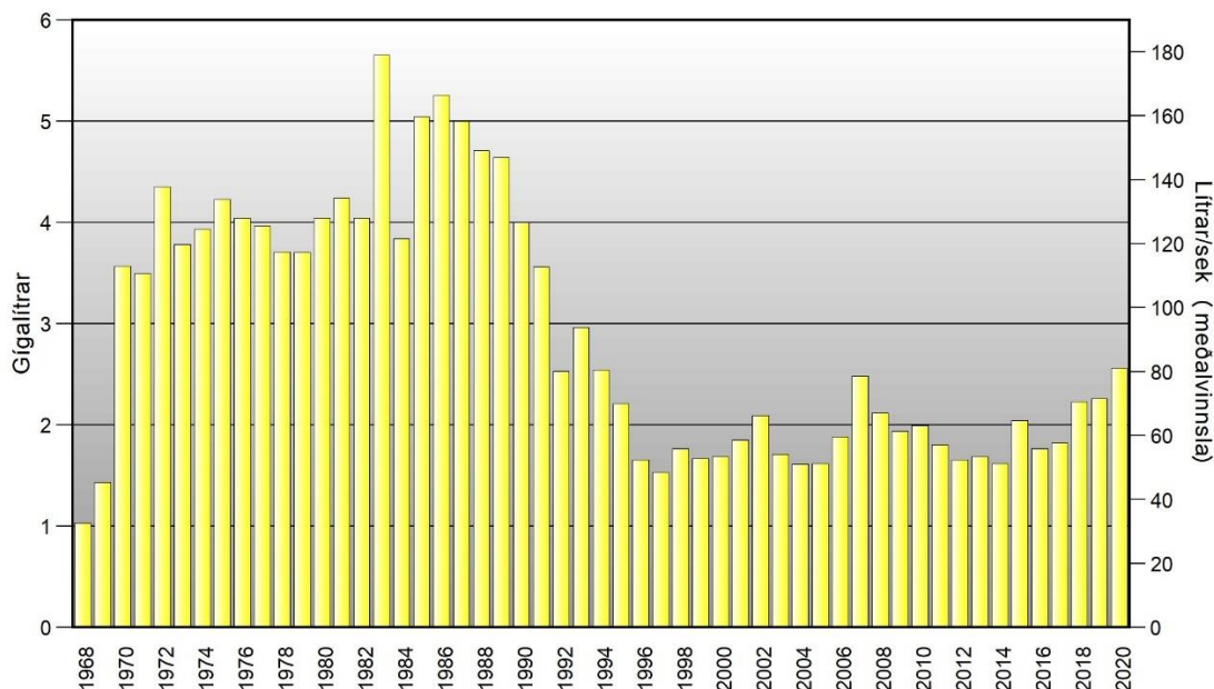
Mynd 16. Árleg heildarvinnsla Elliðaársvæðisins árin 1968 - 2020
