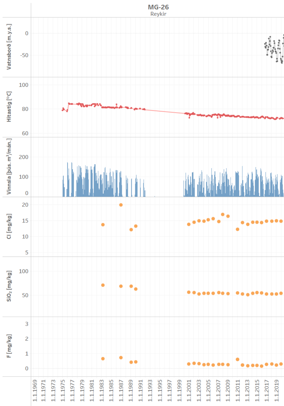
Mynd 46. Vinnsla úr holu MG-26 ásamt breytingum á vatnsborði, hita og efnainnihaldi
