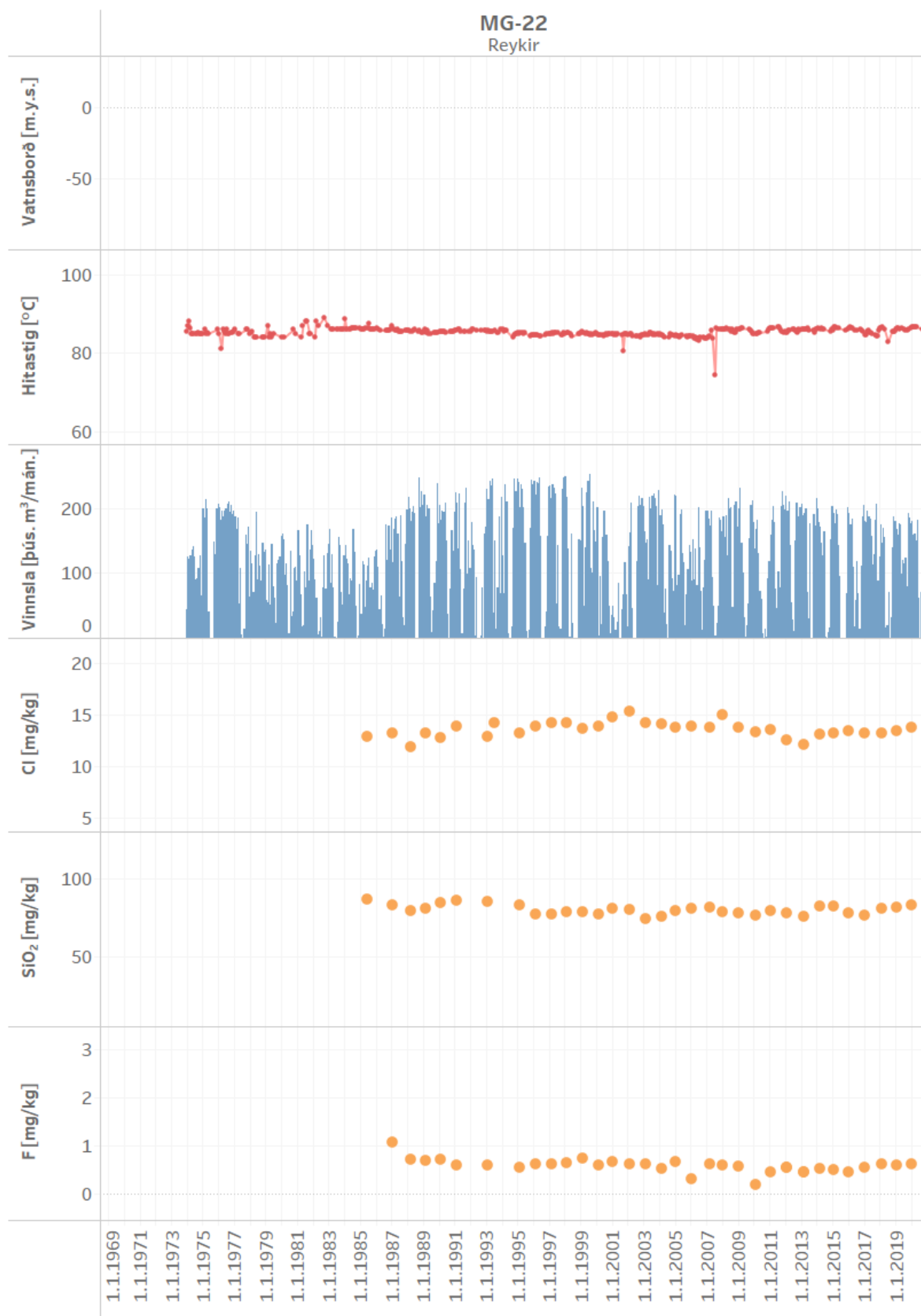
Mynd 42. Vinnsla úr holu MG-22 ásamt breytingum á vatnsborði, hita og efnainnihaldi
