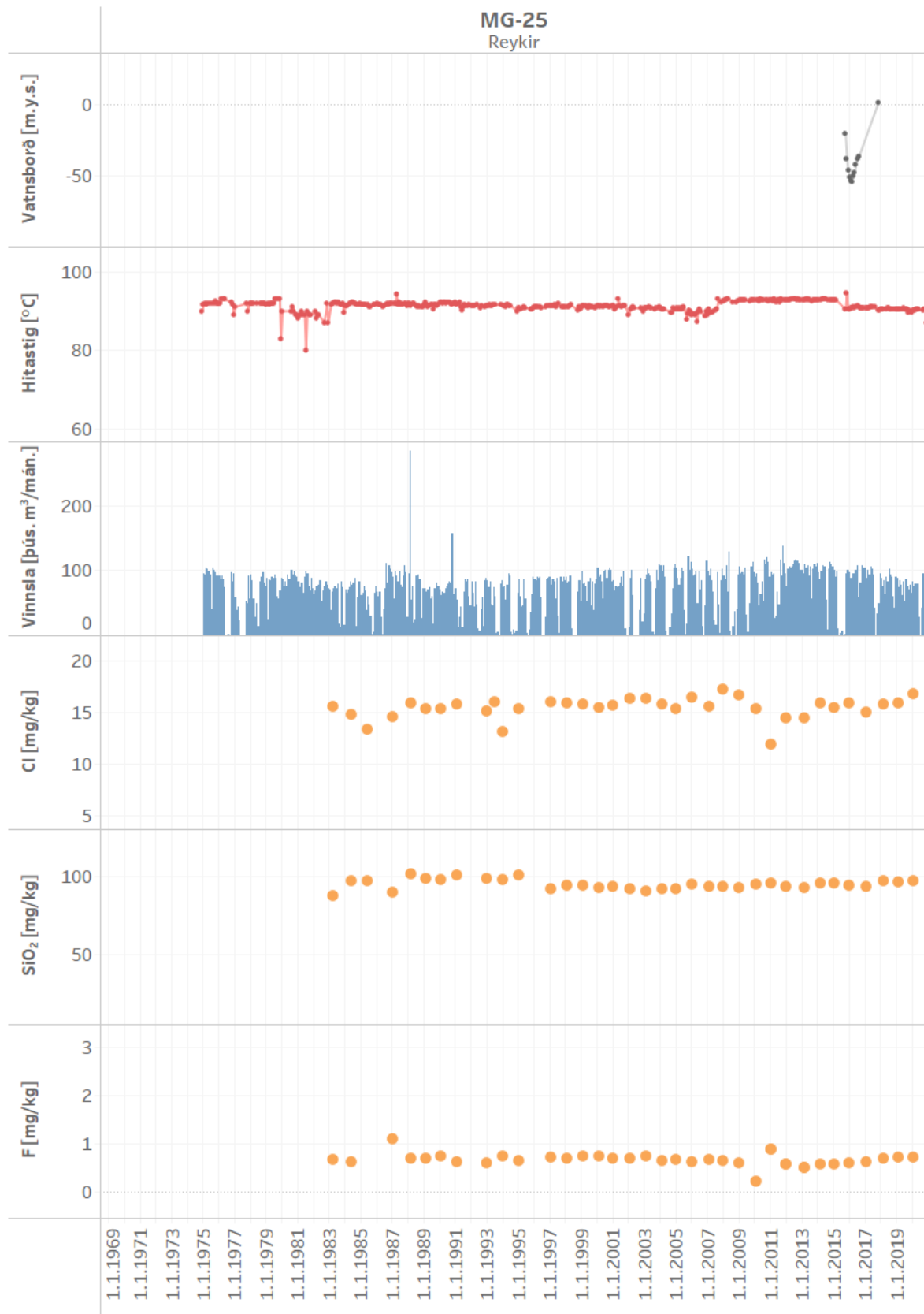
Mynd 45. Vinnsla úr holu MG-25 ásamt breytingum á vatnsborði, hita og efnainnihaldi
