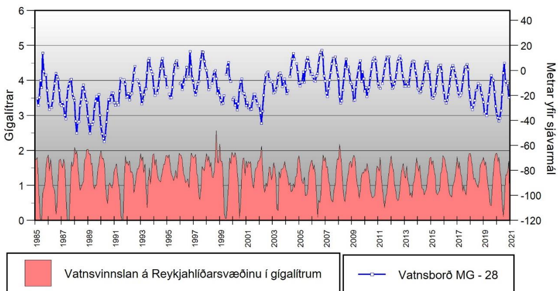
Mynd 51. Mánaðarleg vinnsla í Reykjahlíð árin 1985–2020, ásamt vatnsborði í viðmiðunarholu
