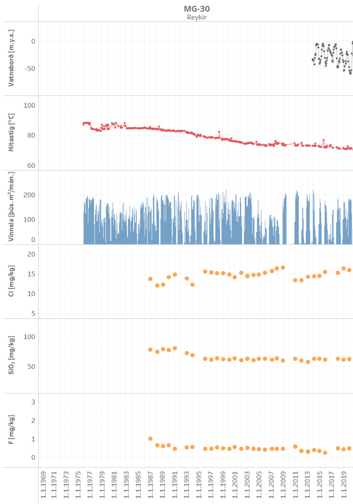
Mynd 48. Vinnsla úr holu MG-30 ásamt breytingum á vatnsborði, hita og efnainnihaldi
