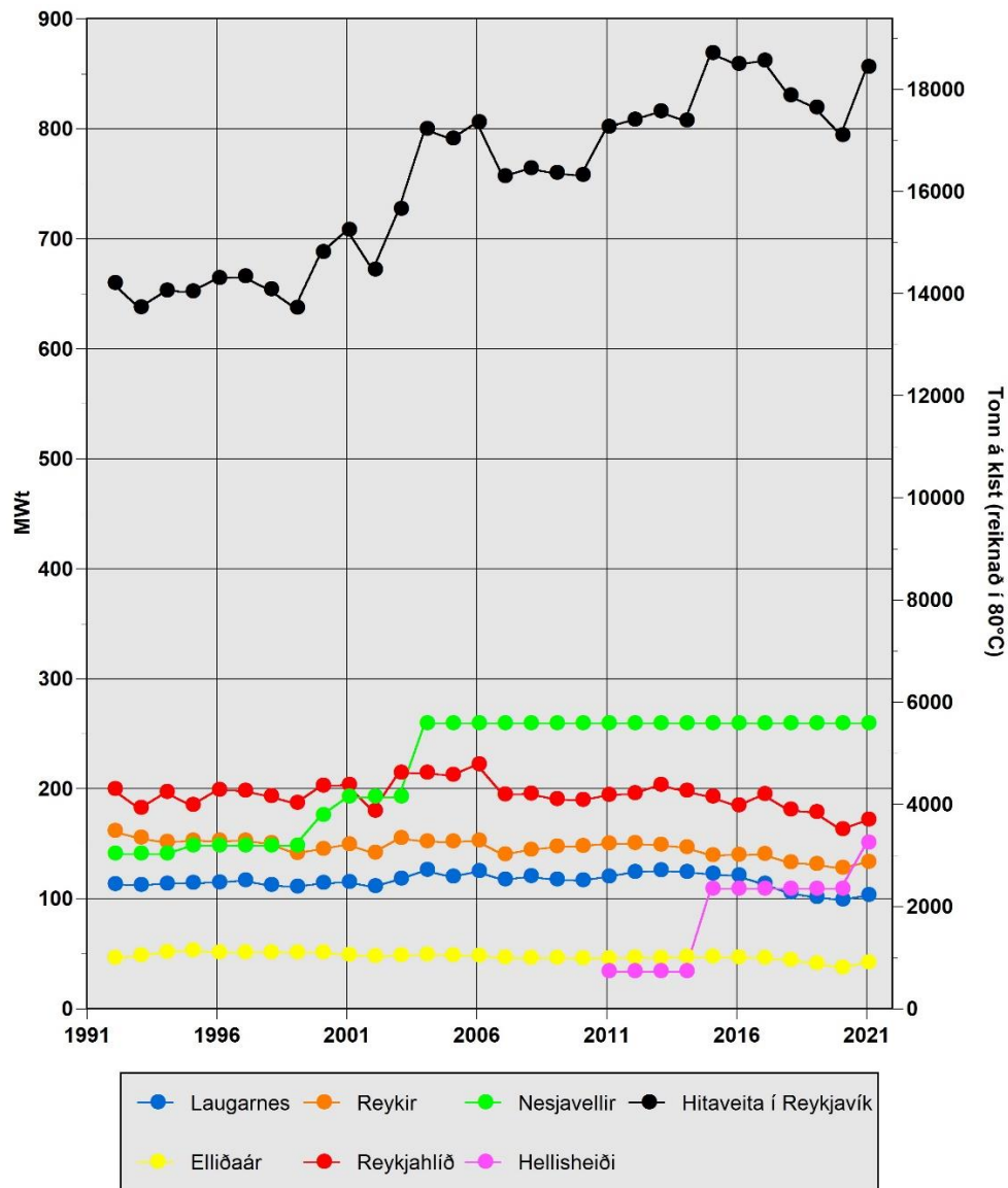
Mynd 3. Breytingar á aflgetu hitaveitu í Reykjavík 1992 – 2021
