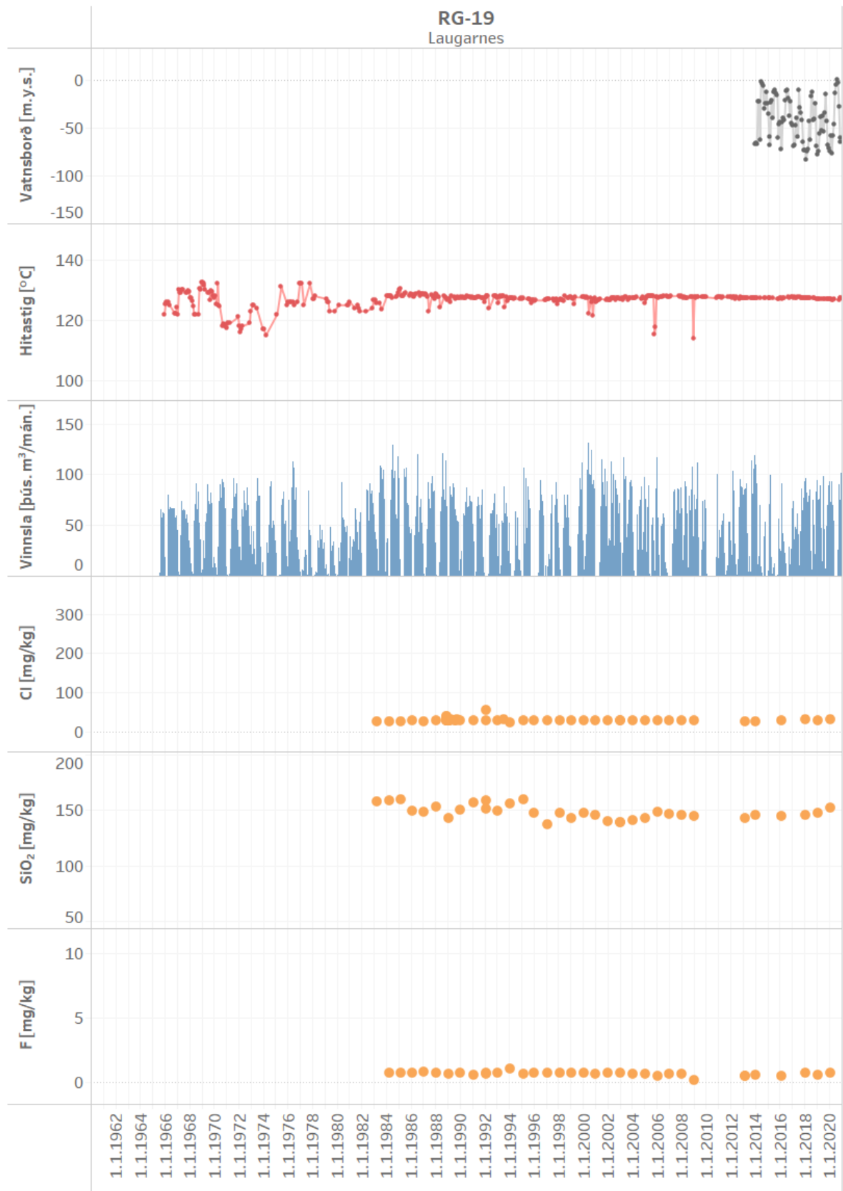
Mynd 12. Vinnsla úr holu RG-19 ásamt breytingum á vatnsborði, hita og efnainnihaldi
