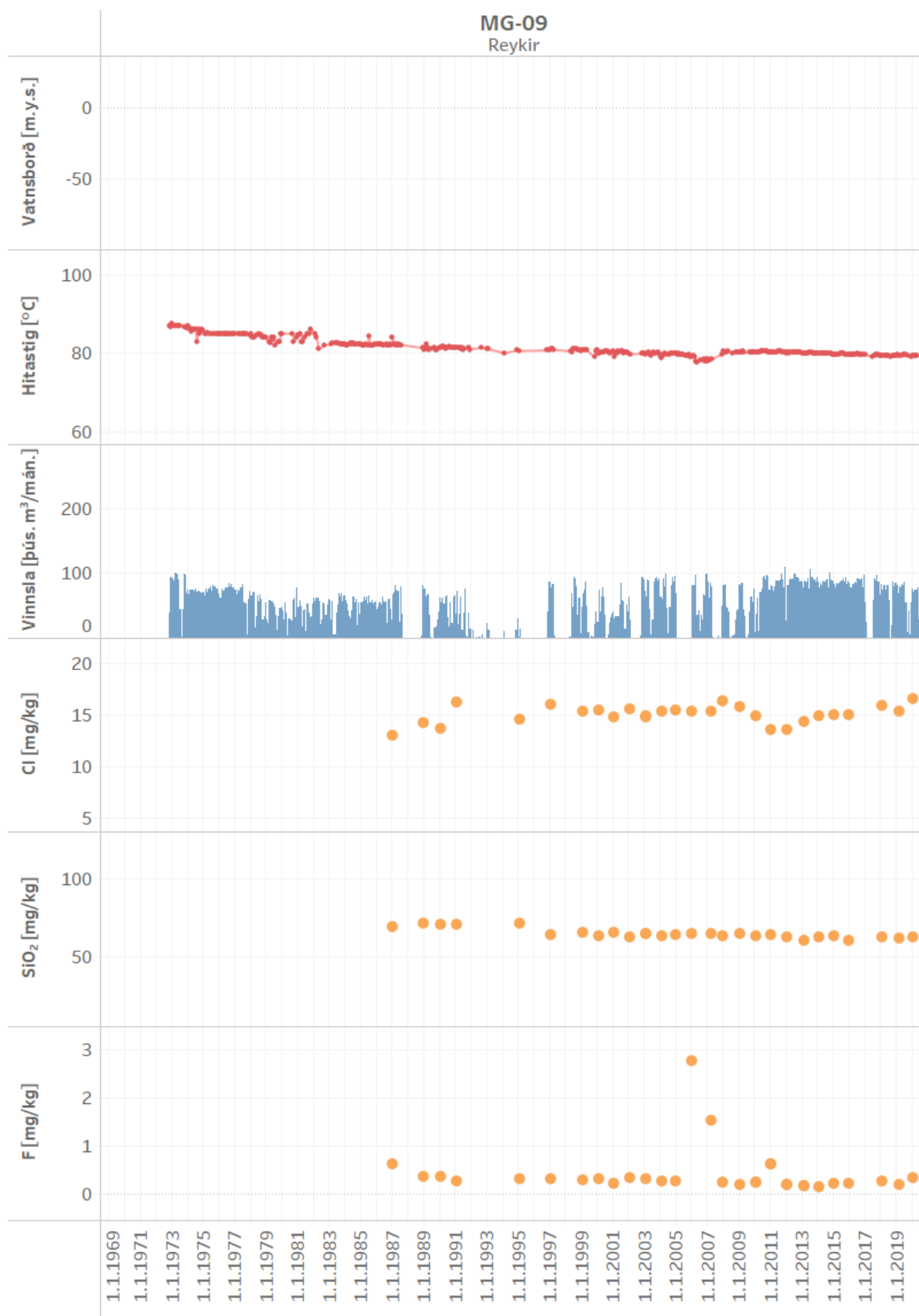
Mynd 32. Vinnsla úr holu MG-09 ásamt breytingum á vatnsborði, hita og efnainnihaldi
