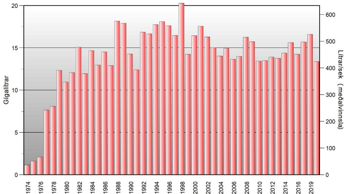
Mynd 50. Árleg heildarvinnsla Reykjahlíðarsvæðisins árin 1974 - 2020
