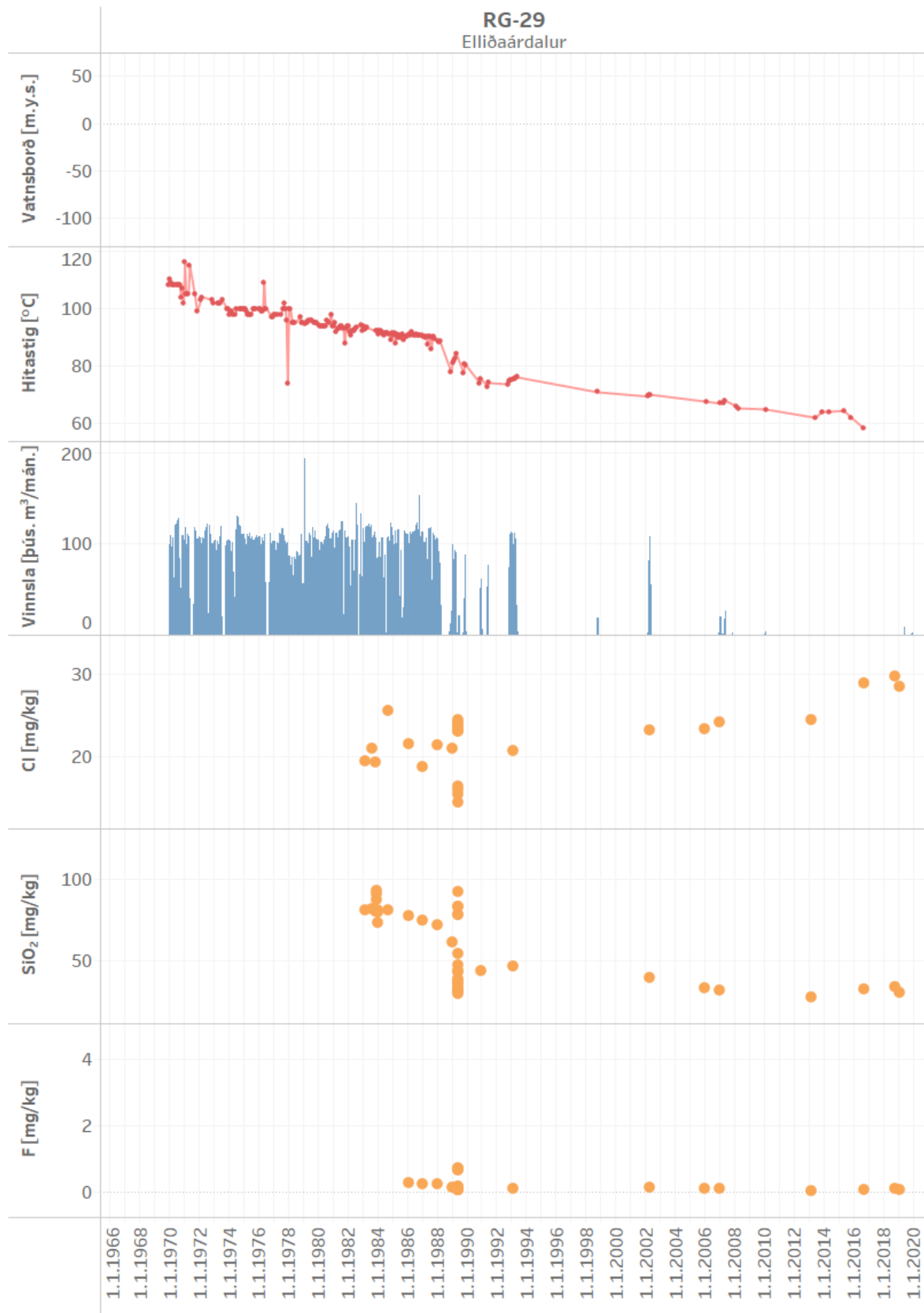
Mynd 20. Vinnsla úr holu RG-29 ásamt breytingum á vatnsborði, hita og efnainnihaldi
