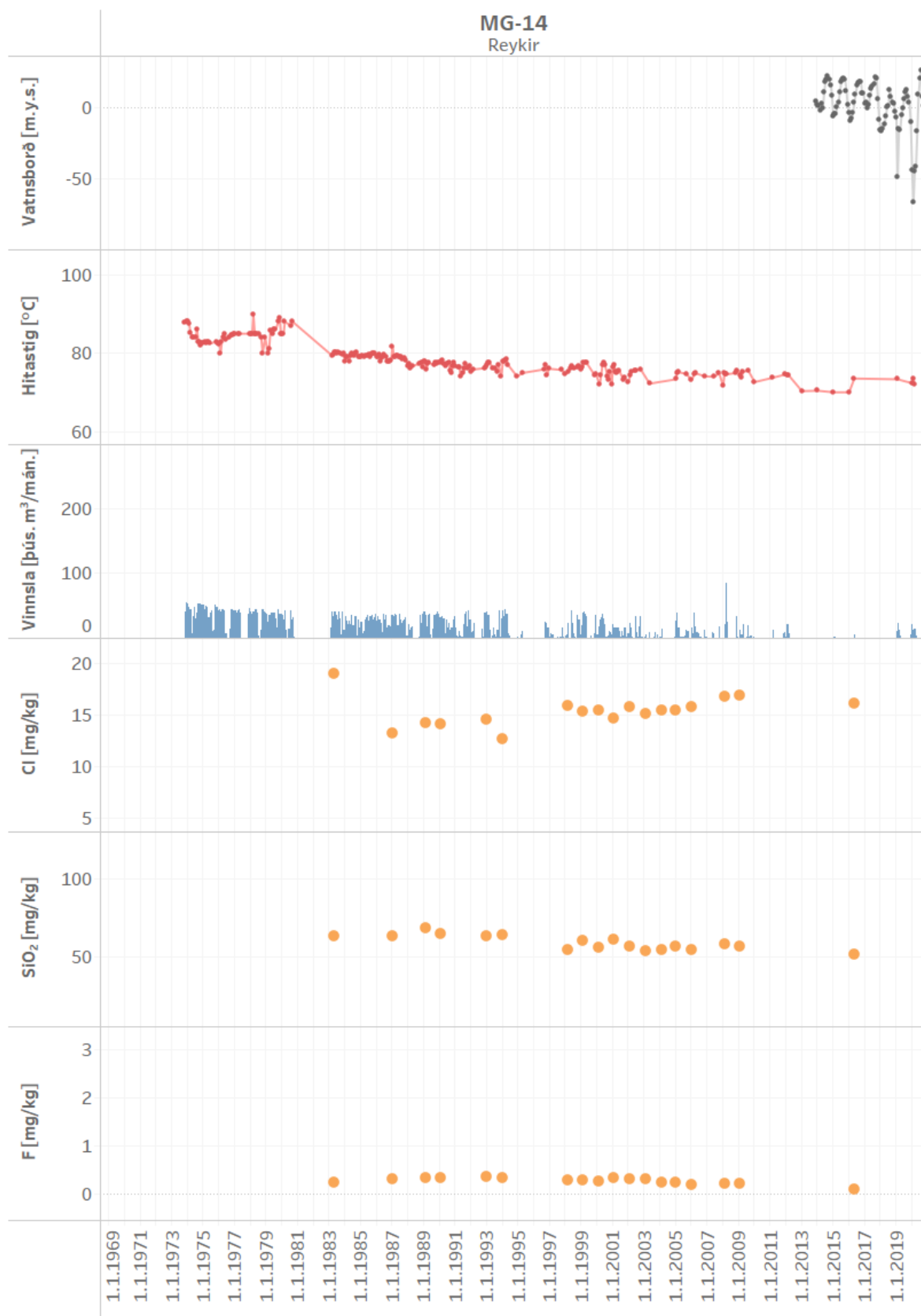
Mynd 36. Vinnsla úr holu MG-14 ásamt breytingum á vatnsborði, hita og efnainnihaldi
