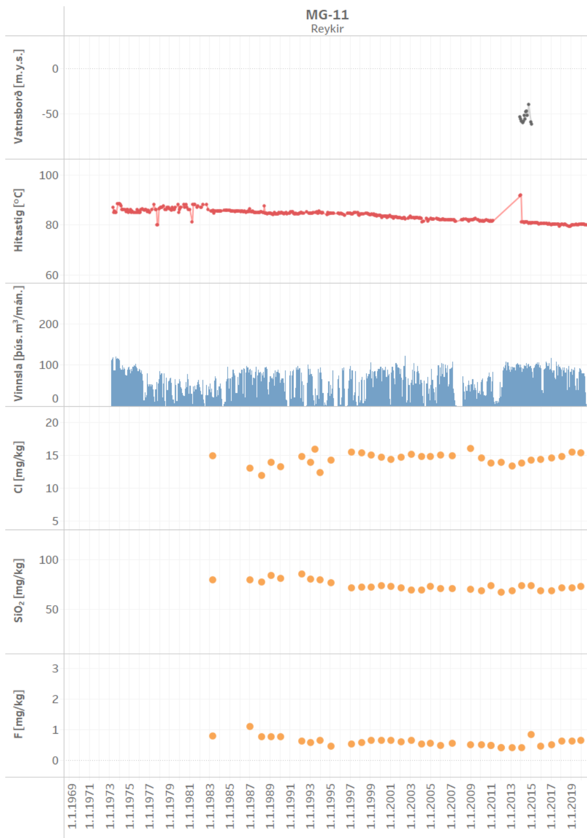
Mynd 33. Vinnsla úr holu MG-11 ásamt breytingum á vatnsborði, hita og efnainnihaldi
