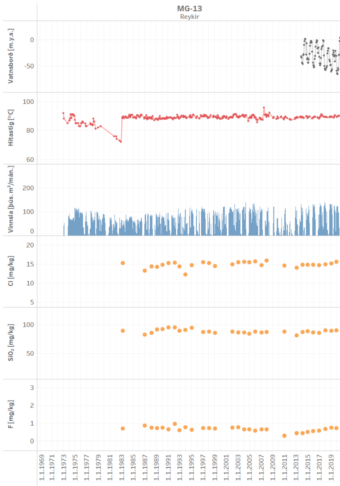
Mynd 35. Vinnsla úr holu MG-13 ásamt breytingum á vatnsborði, hita og efnainnihaldi
