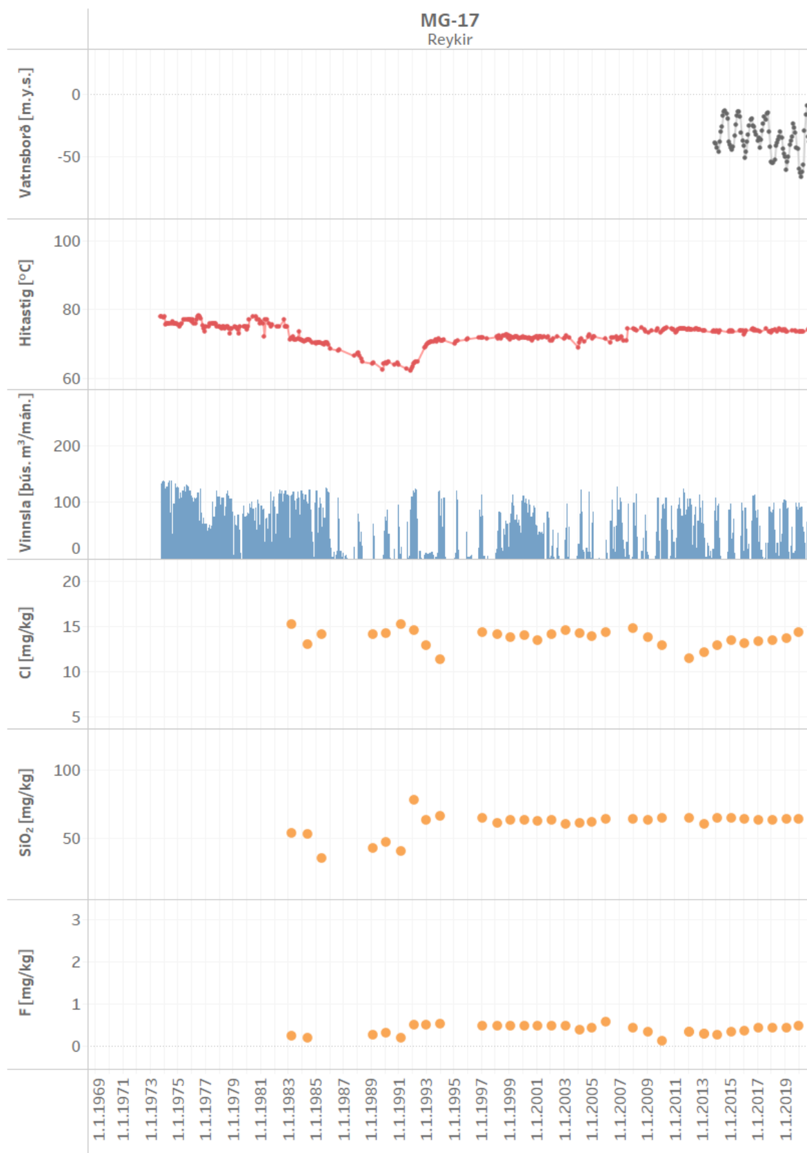
Mynd 39. Vinnsla úr holu MG-17 ásamt breytingum á vatnsborði, hita og efnainnihaldi
