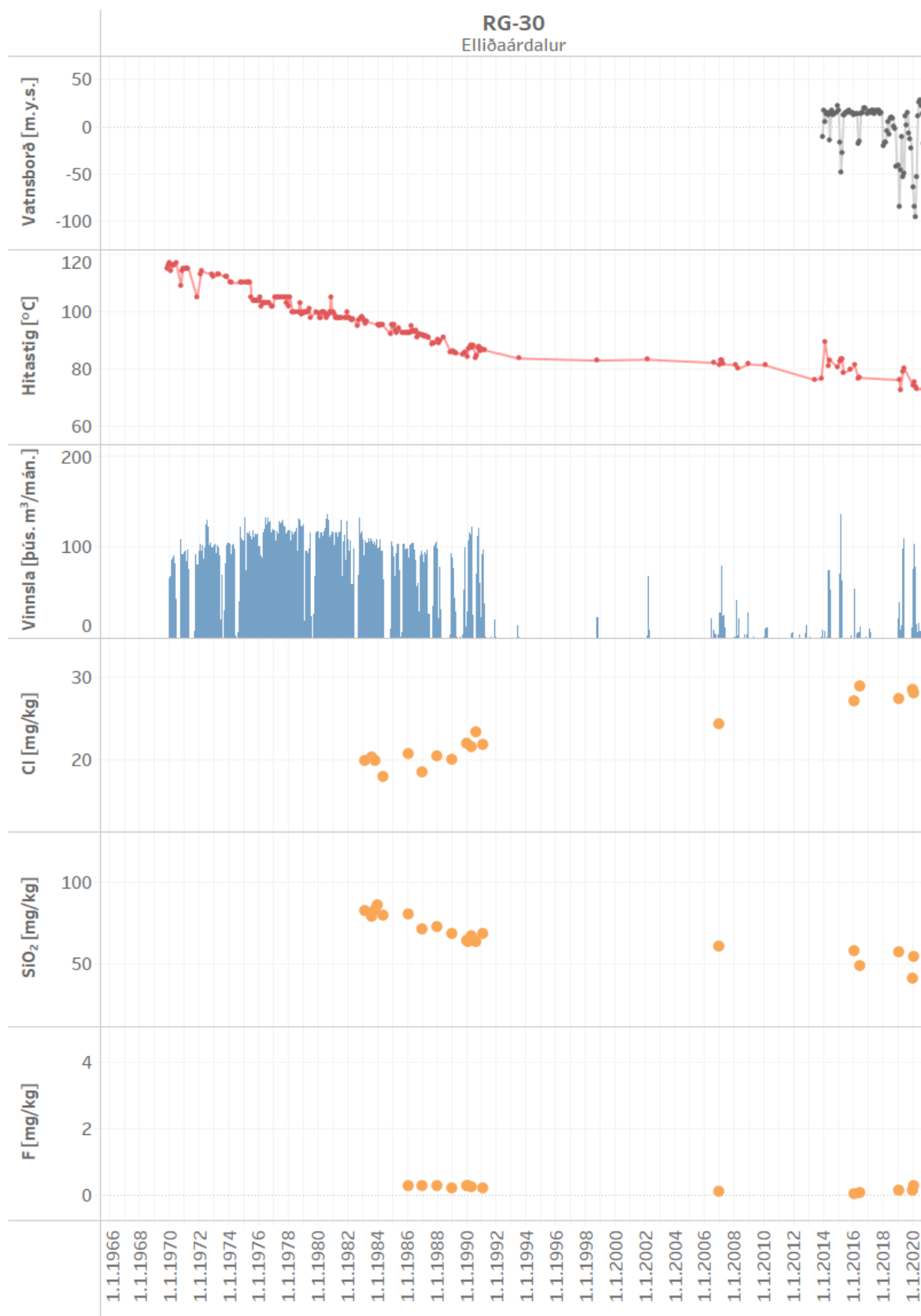
Mynd 21. Vinnsla úr holu RG-30 ásamt breytingum á vatnsborði, hita og efnainnihaldi
