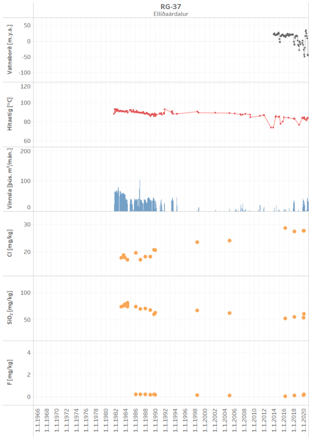
Mynd 24. Vinnsla úr holu RG-37 ásamt breytingum á vatnsborði, hita og efnainnihaldi
