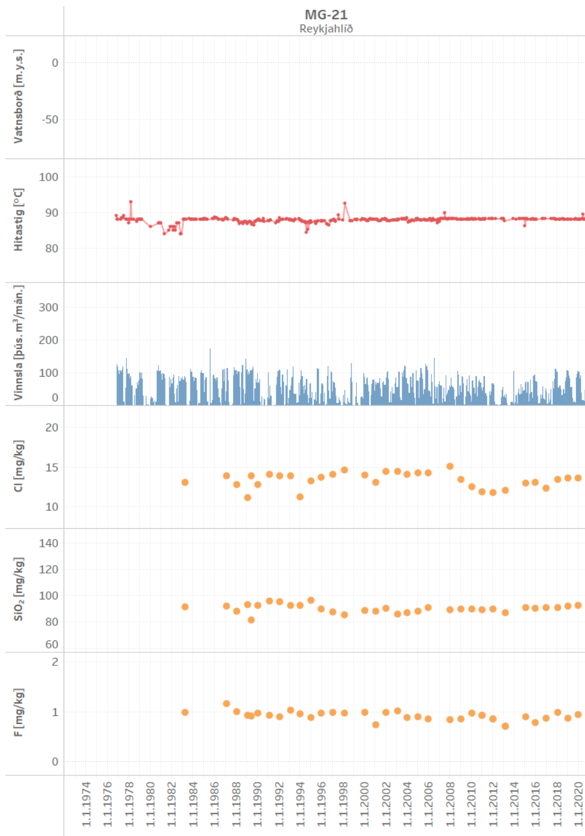
Mynd 54. Vinnsla úr holu MG-21 ásamt breytingum á vatnsborði, hita og efnainnihaldi
