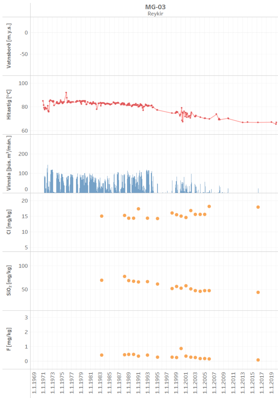
Mynd 28. Vinnsla úr holu MG-03 ásamt breytingum á vatnsborði, hita og efnainnihaldi
