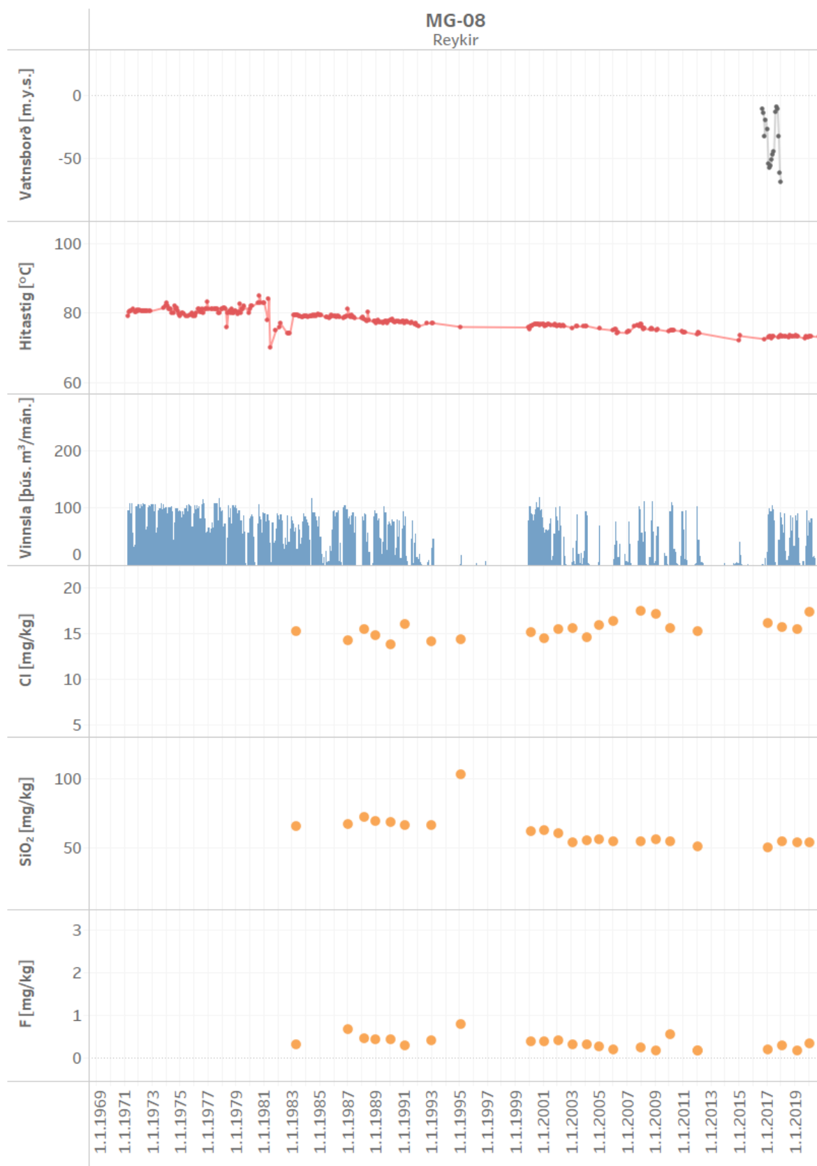
Mynd 31. Vinnsla úr holu MG-08 ásamt breytingum á vatnsborði, hita og efnainnihaldi
