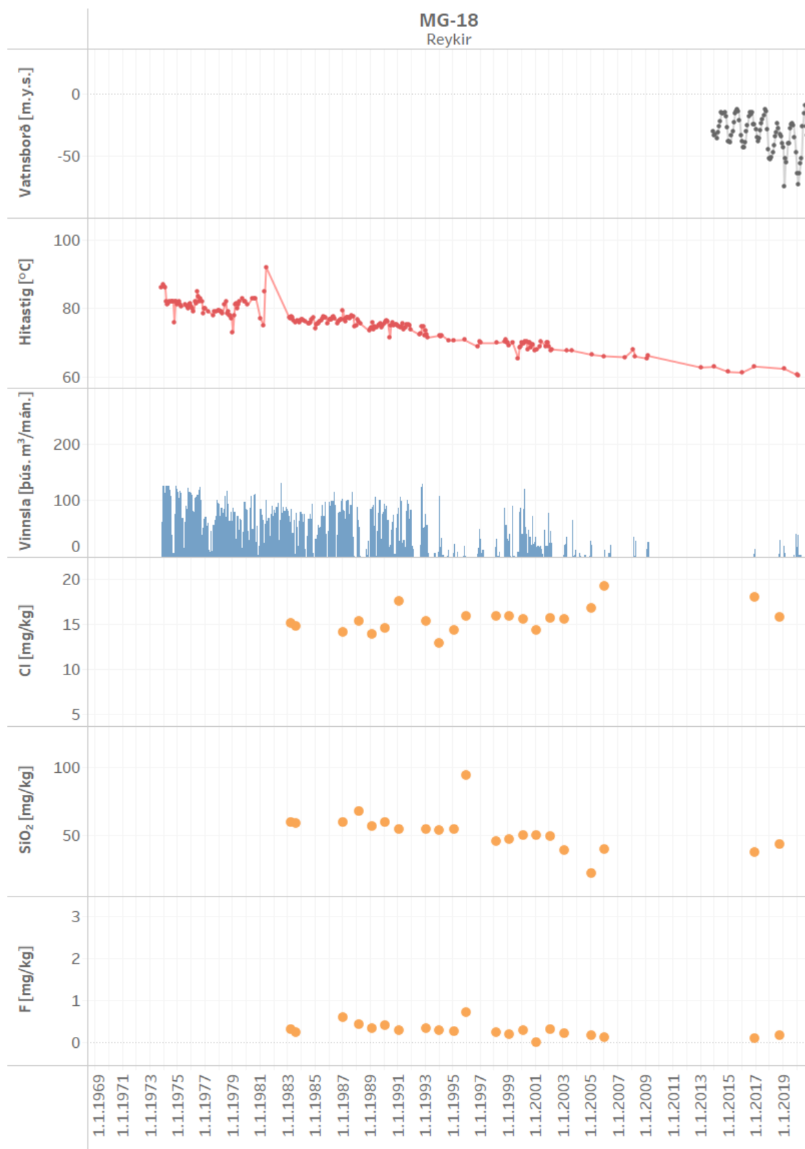
Mynd 40. Vinnsla úr holu MG-18 ásamt breytingum á vatnsborði, hita og efnainnihaldi
