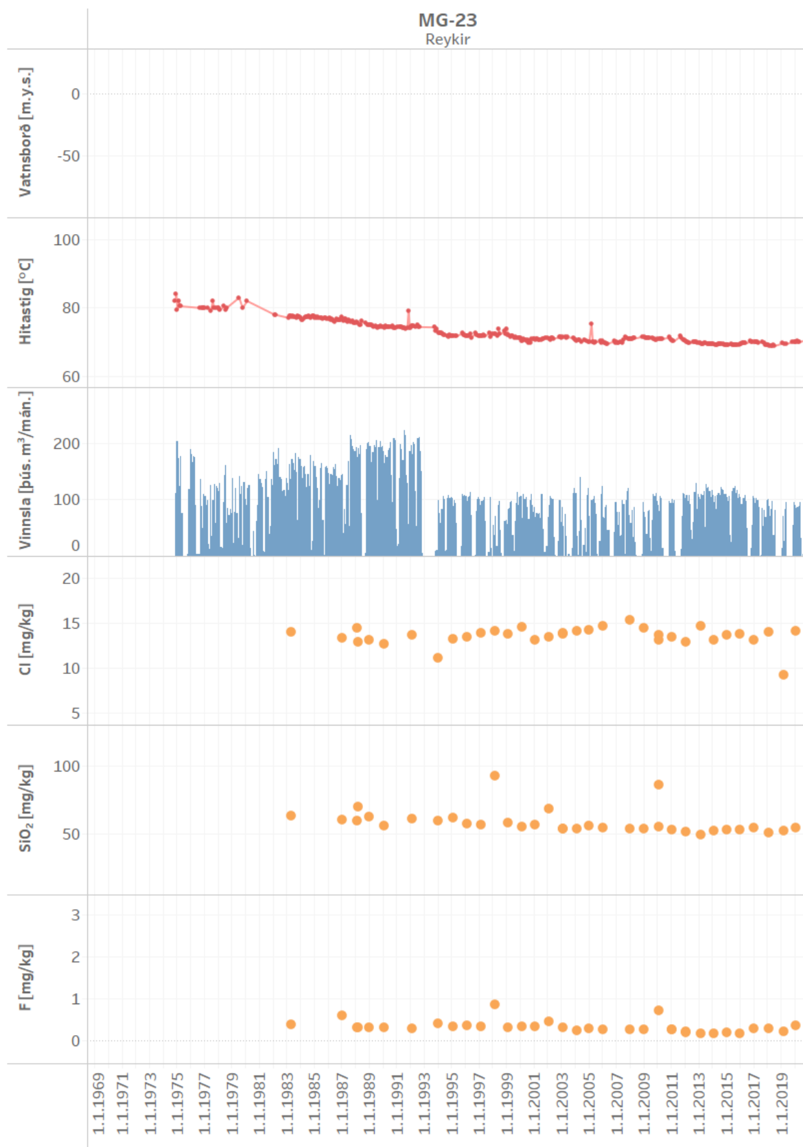
Mynd 43. Vinnsla úr holu MG-23 ásamt breytingum á vatnsborði, hita og efnainnihaldi
