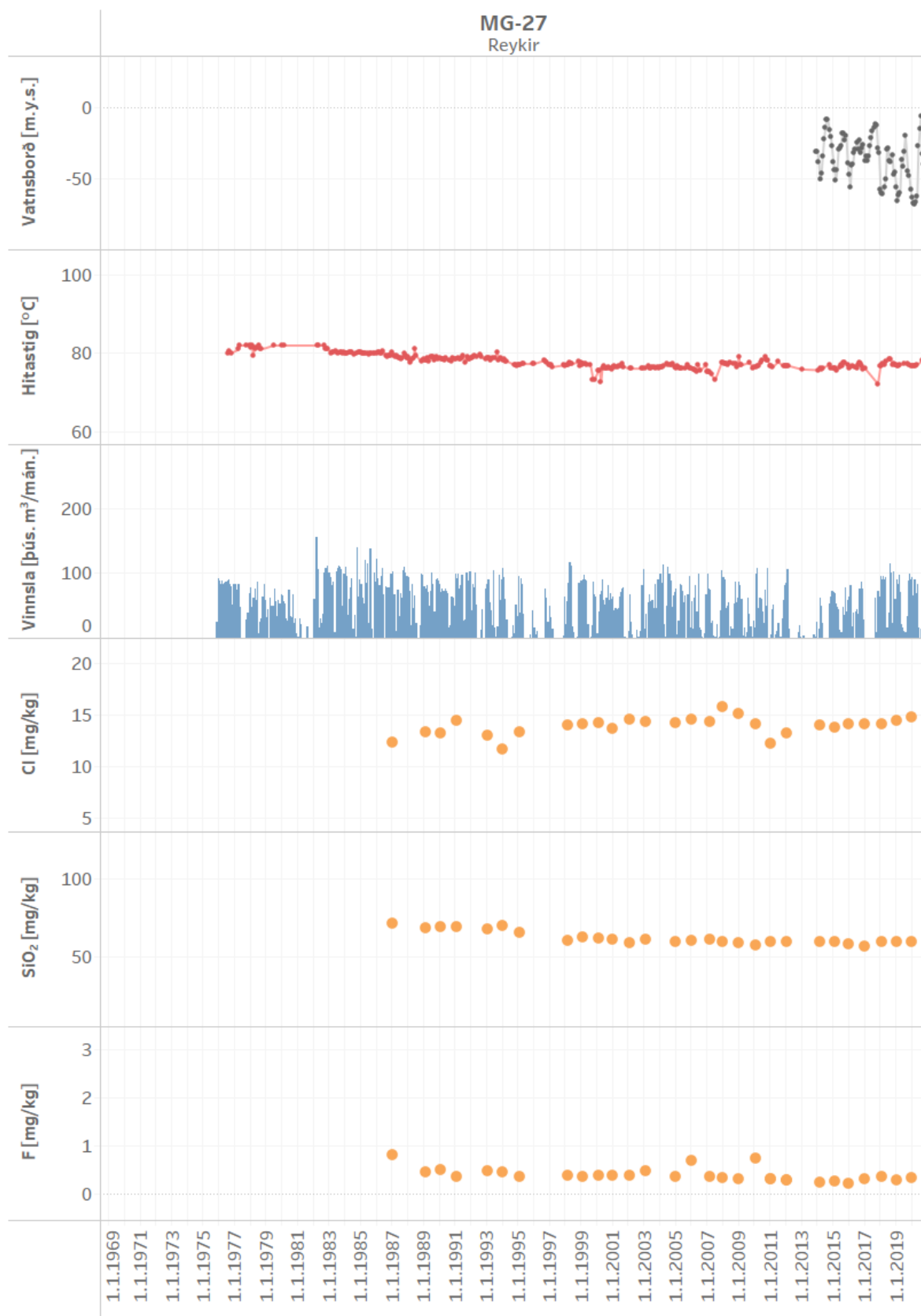
Mynd 47. Vinnsla úr holu MG-27 ásamt breytingum á vatnsborði, hita og efnainnihaldi
