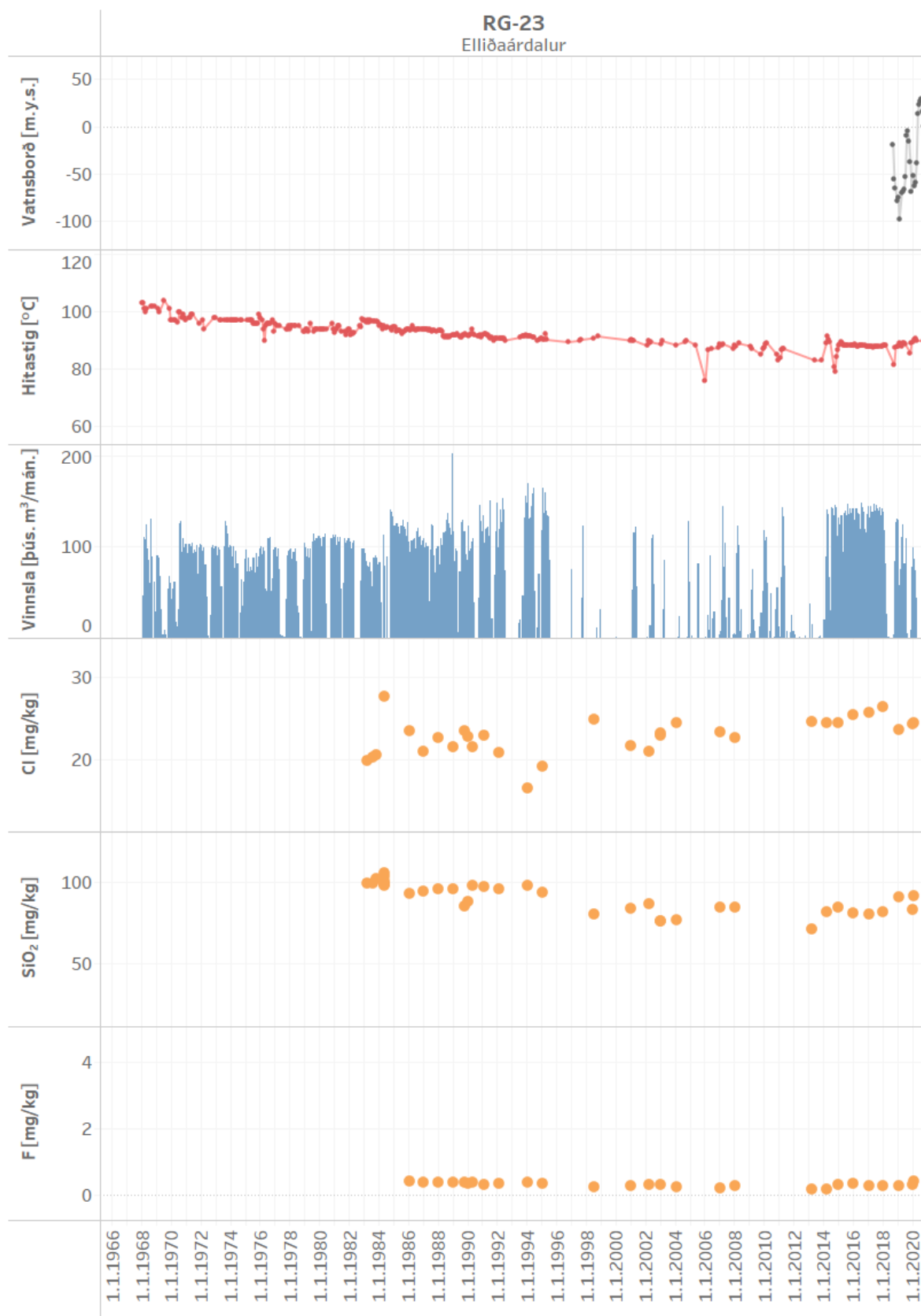
Mynd 18. Vinnsla úr holu RG-23 ásamt breytingum á vatnsborði, hita og efnainnihaldi
