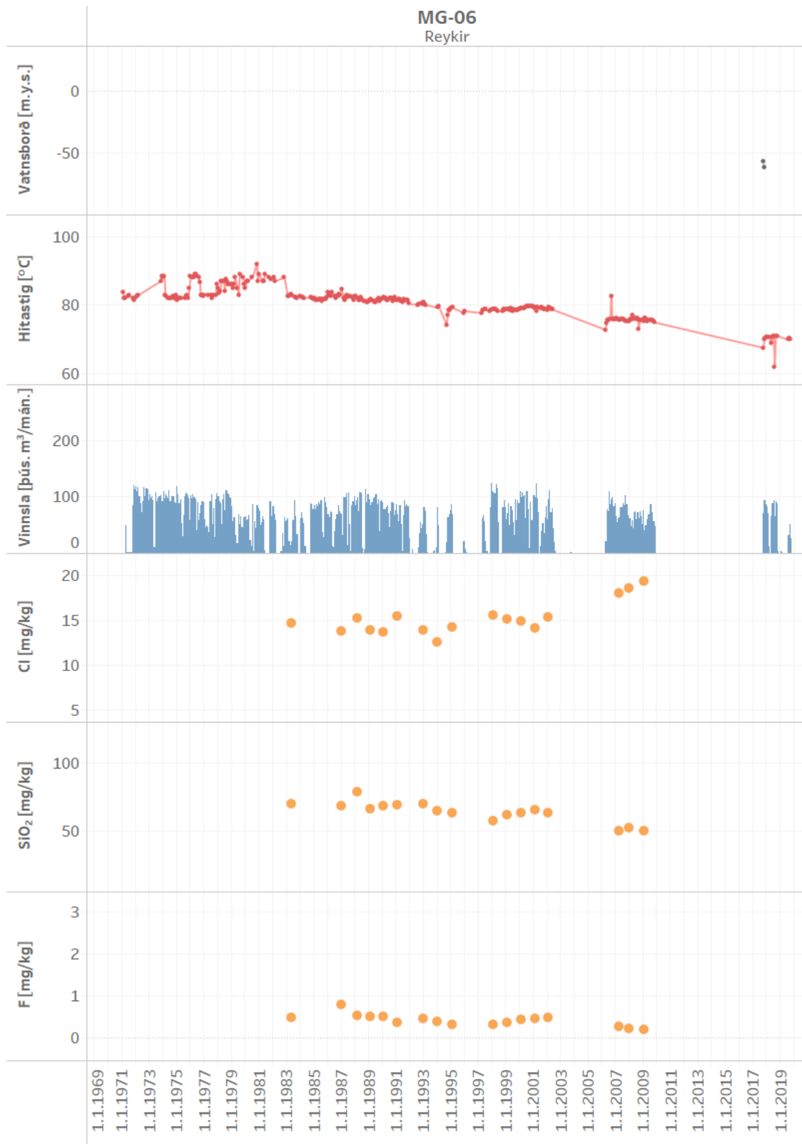
Mynd 30. Vinnsla úr holu MG-06 ásamt breytingum á vatnsborði, hita og efnainnihaldi
