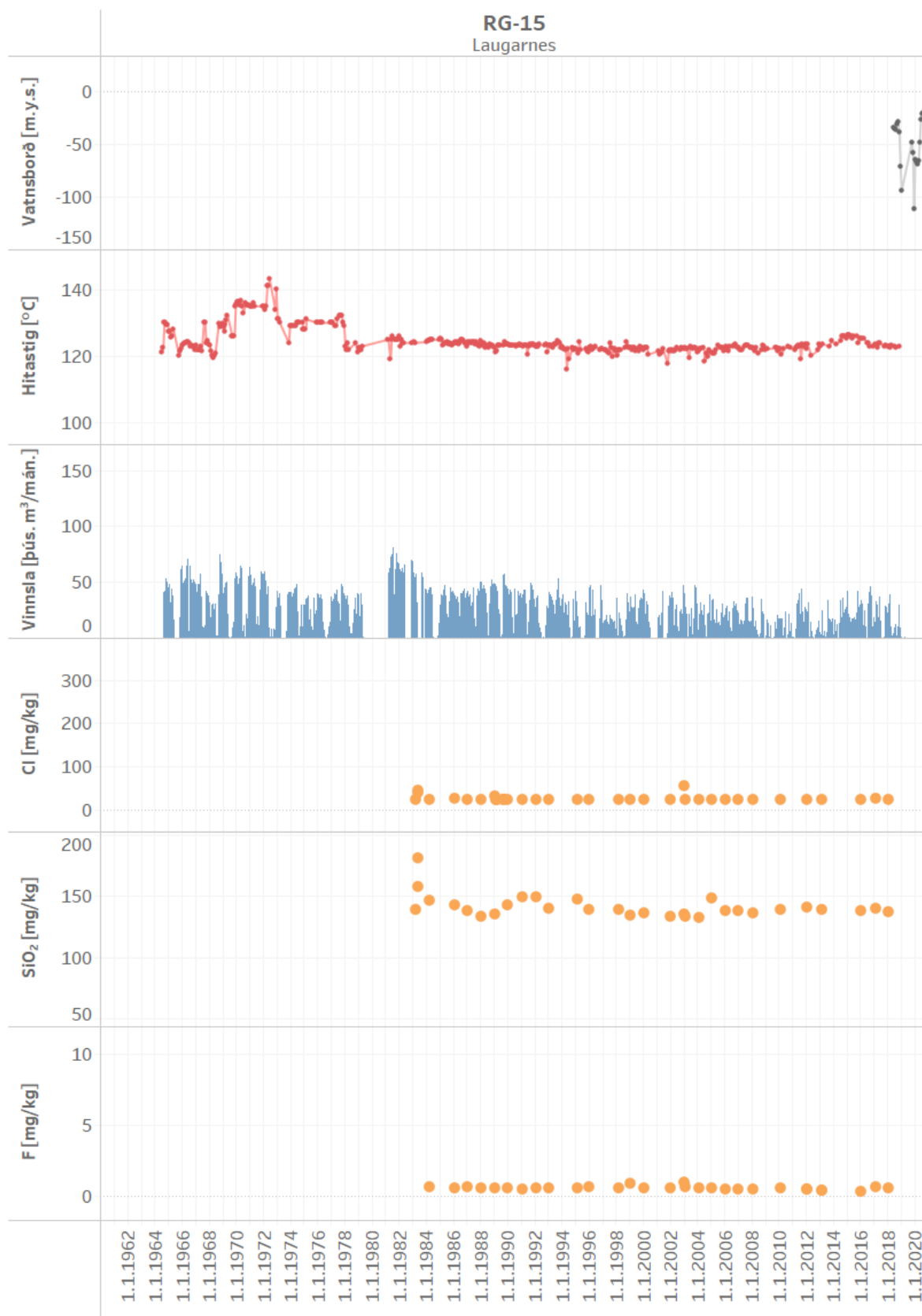
Mynd 10. Vinnsla úr holu RG-15 ásamt breytingum á vatnsborði, hita og efnainnihaldi
