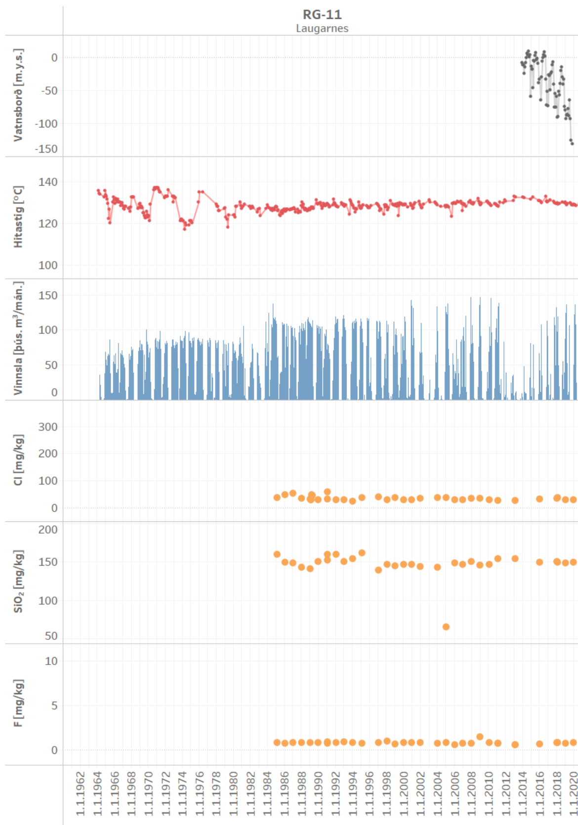
Mynd 9. Vinnsla úr holu RG-11 ásamt breytingum á vatnsborði, hita og efnainnihaldi
