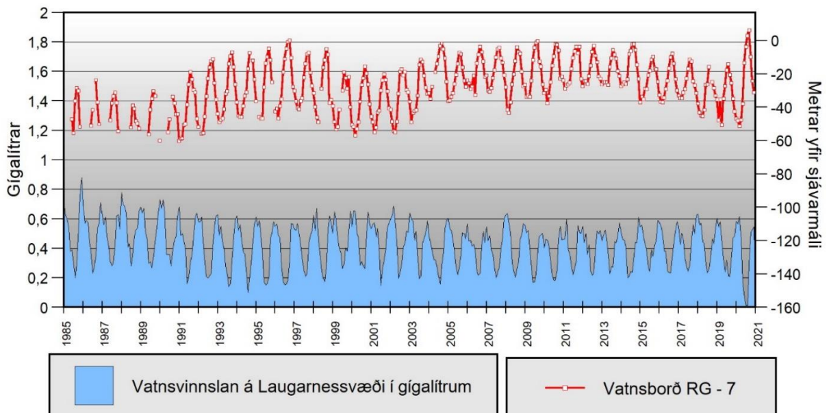
Mynd 5. Mánaðarleg vinnsla á Laugarnesi árin 1985–2020, ásamt vatnsborði í viðmiðunarholu
