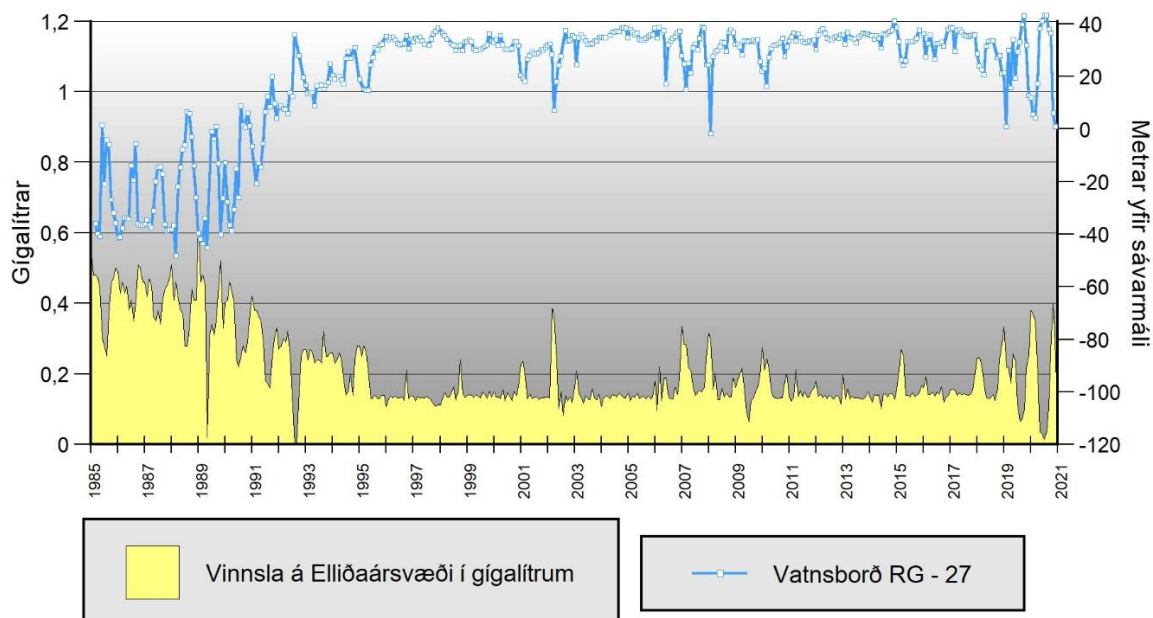
Mynd 17. Mánaðarleg vinnsla í Elliðaá 1985–2020, ásamt vatnsborði í viðmiðunarholu
