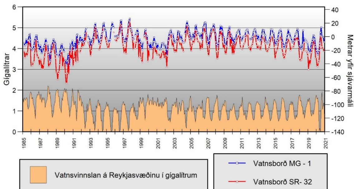
Mynd 27. Mánaðarleg vinnsla á Reykjum árin 1985–2020, ásamt vatnsborði í viðmiðunarholum
