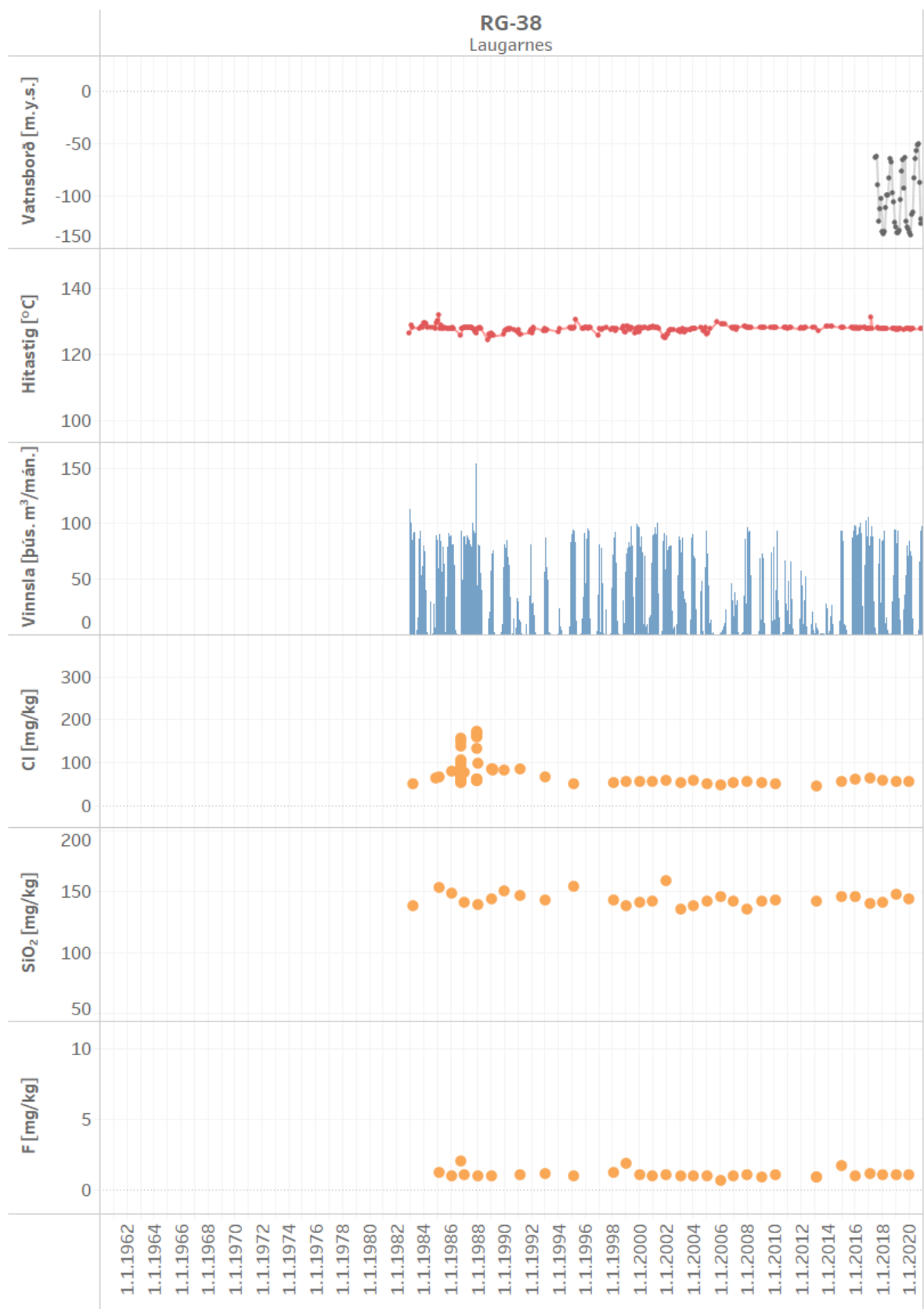
Mynd 15. Vinnsla úr holu RG-38 ásamt breytingum á vatnsborði, hita og efnainnihaldi
