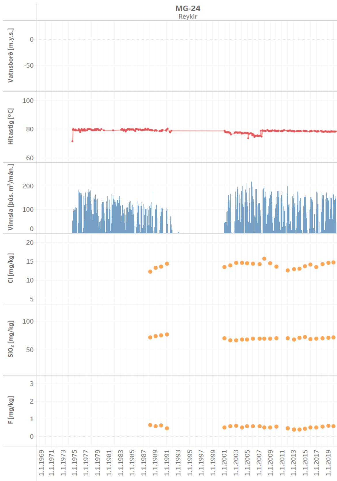
Mynd 44. Vinnsla úr holu MG-24 ásamt breytingum á vatnsborði, hita og efnainnihaldi
