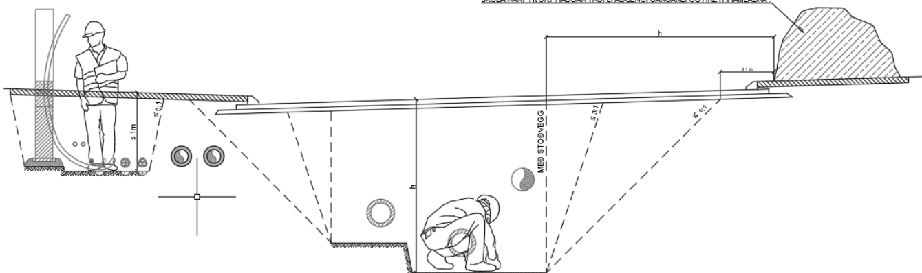
Mynd 13: Öryggi við skurðgröft og gryfjur (LAV-131)
