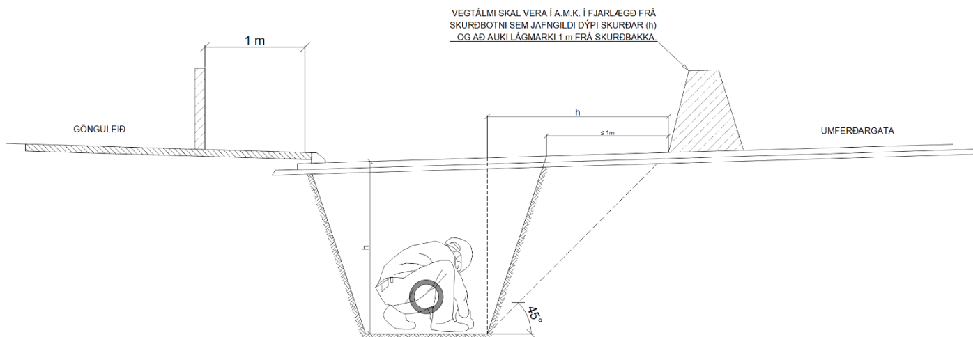
Mynd 14: Fjarlægð vegtálma og girðinga frá skurði
