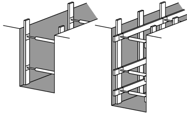
Mynd 11: Dæmi um stoðir
