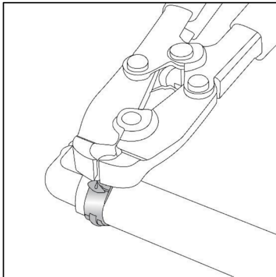
3. Полностью разрежьте и снимите хомут
