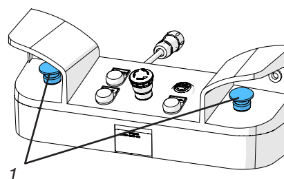
Fig. 44: Butoane de declanșare Operare cu 2 mâini
