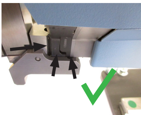
Fig. 54: SKS Senzor de tracțiune cu poziționare corectă
