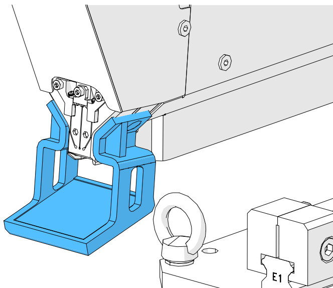
Fig. 107: Verificarea fălcilor de sertizare cu oglinda de testare a fălcilor montate
