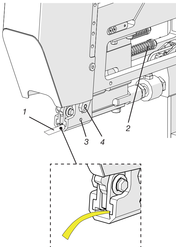
Fig. 131: Setarea senzorului de detectare a benzii
