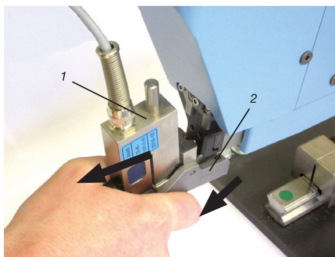
Fig. 56: Forța de tracțiune de verificare
