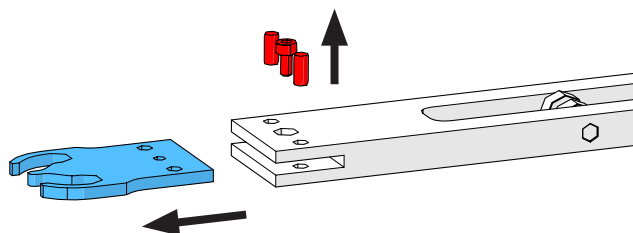
Fig. 125: Pană de sertizare
