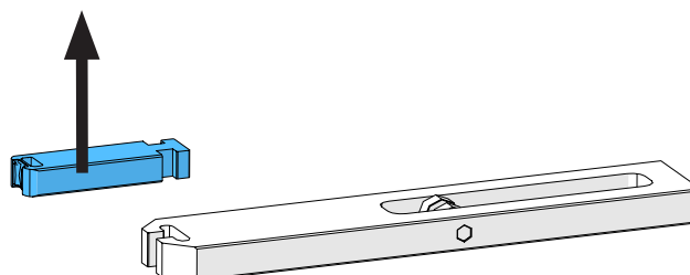
Fig. 123: Dezasamblat, separând poansonul separator și glisorul
