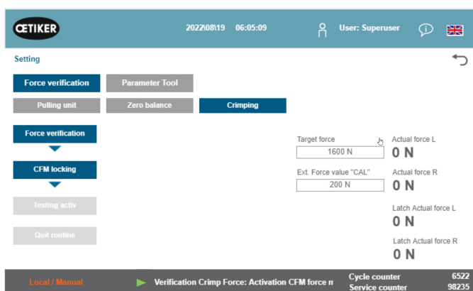
Fig. 57: Verificarea forței de sertizare
