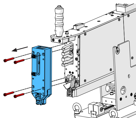
Fig. 115: Cap de dezasamblare
