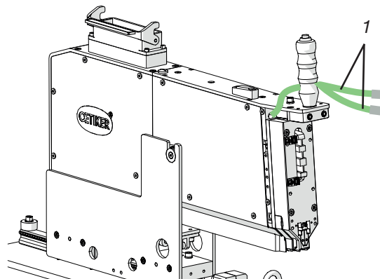
Fig. 114: Senzori de monitorizare a sertizării
