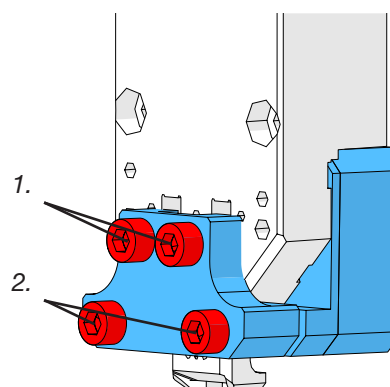
Fig. 126: Dispozitiv de introducere/scoatere prin presare
