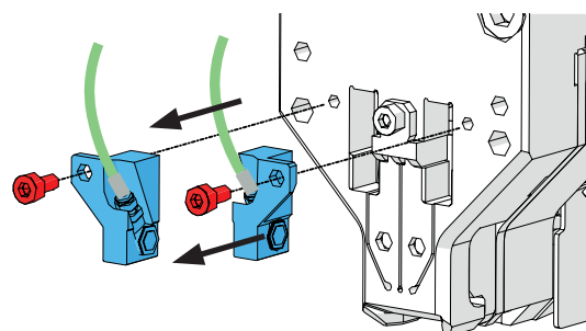
Fig. 113: Demontare senzori de monitorizare a sertizării
