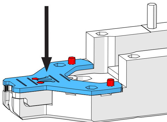
Fig. 122: Placă de distanțare pentru montare
