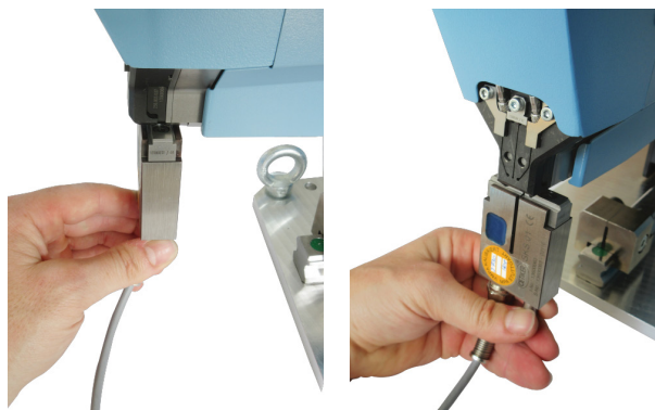
Fig. 58: Poziționarea forței de sertizare SKS
