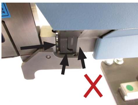
Fig. 55: Poziționare incorectă a senzorului de tracțiune SKS
