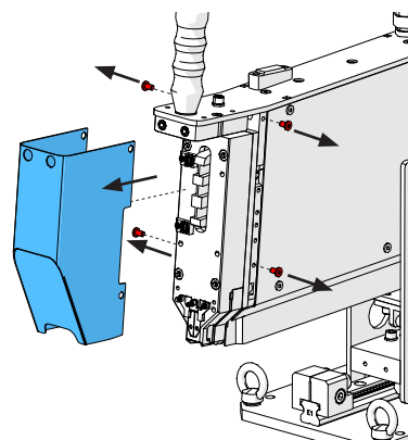
Fig. 112: Demontarea capului de protecție
