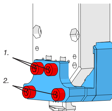
Fig. 127: Dispozitiv de introducere/scoatere prin presare
