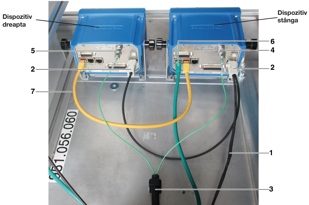
Fig. 24: Unitate de control, conexiuni
