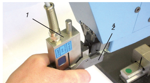
插图 53: SKS 拉力传感器
