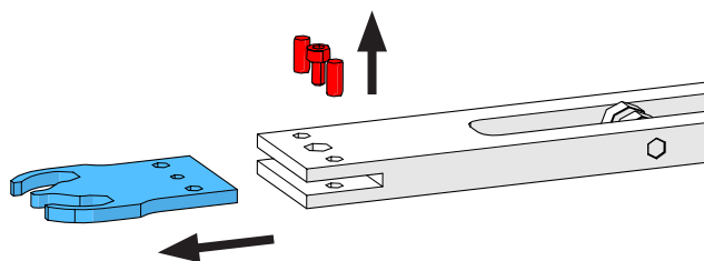
插图 121: 夹紧楔形件
