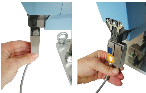
插图 57: 验证压接力
