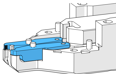
插图 117: 装配夹紧钳
