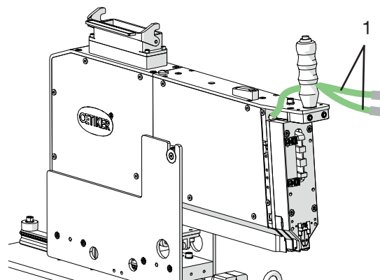
插图 110: 夹紧监测传感器
