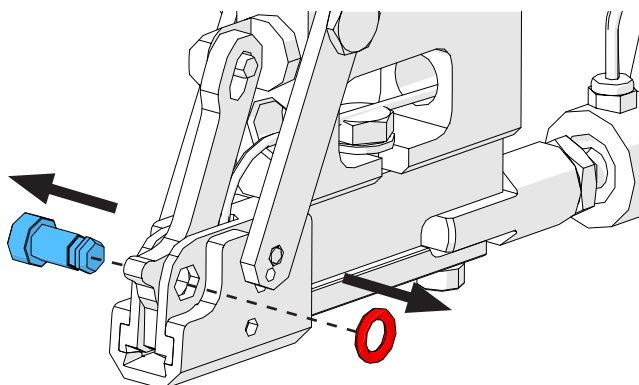
插图 124: 拆卸夹紧杆
