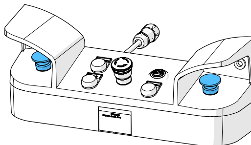
插图 46: 释放按钮, 双手操作
