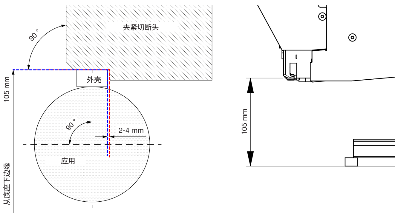
插图 40: 校准工具
