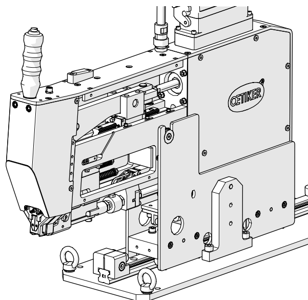
插图 123: 已拆下前盖板的工具
