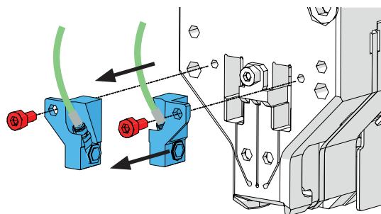
插图 109: 拆卸夹紧监测传感器
