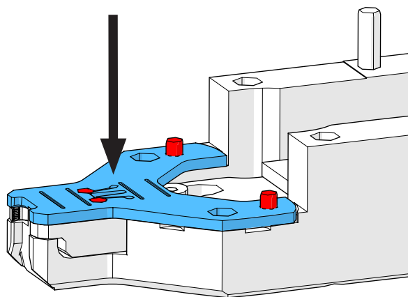
插图 118: 安装垫板
