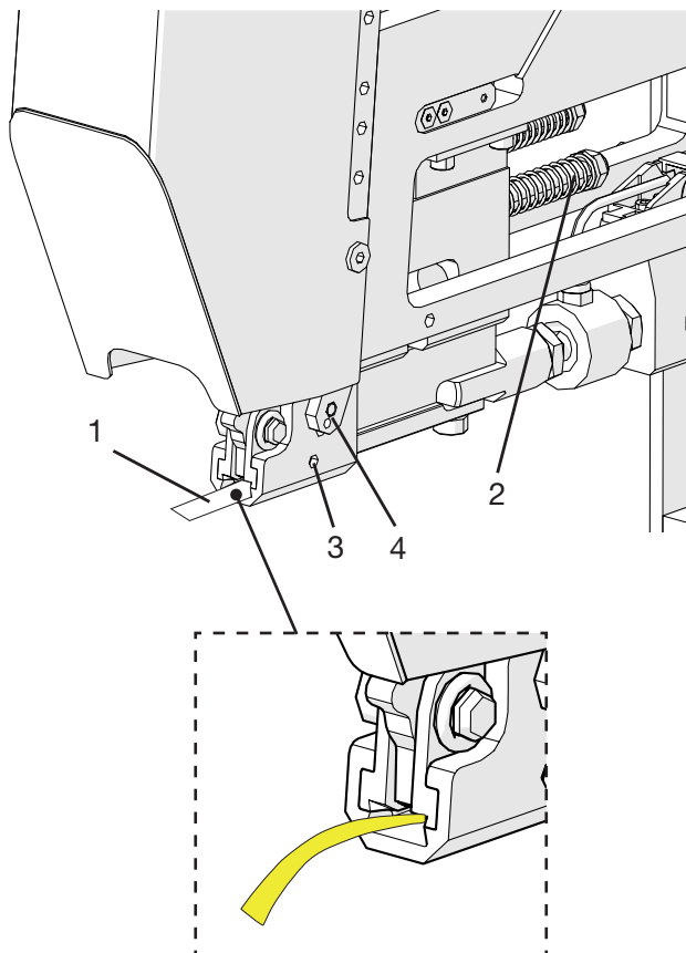
插图 126: 设置条带检测传感器
