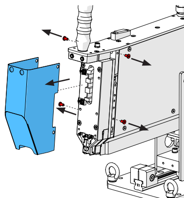
插图 108: 拆卸保护盖板头
