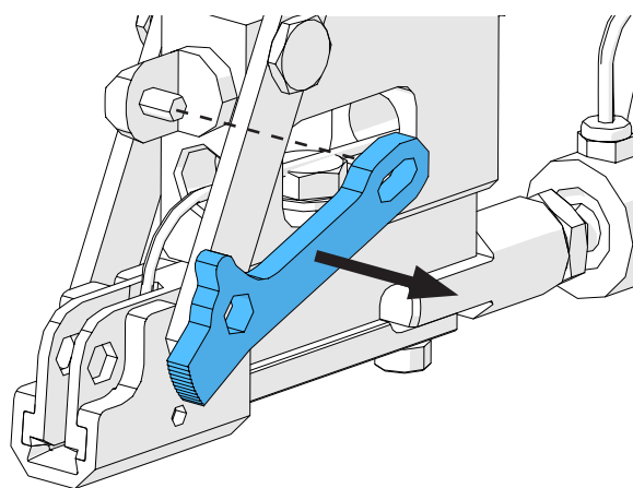
插图 125: 夹紧杆
