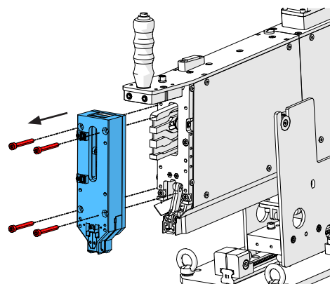
插图 110: 夹紧监测传感器
