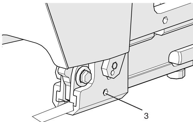
插图 127: 设置条带检测传感器
