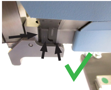
插图 54: SKS 正确定位拉力传感器
