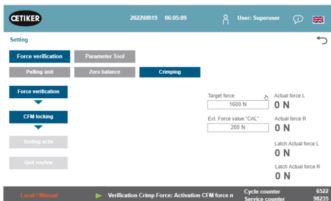
插图 57: 验证压接力
