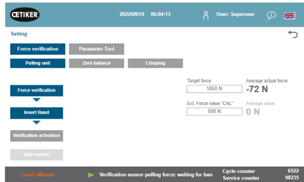
插图 52: 验证张紧力
