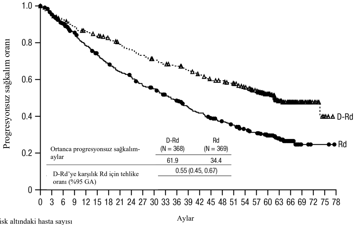
Şekil 1: MMY3008 çalışmasında Kaplan-Meier PFS eğrisi
