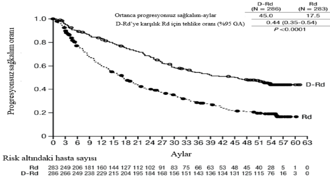
Şekil 6: MMY3003 çalışmasında PFS'nin Kaplan-Meier eğrisi
