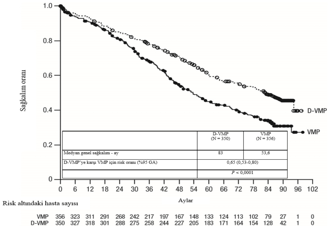
Şekil 4: MMY3007 çalışmasında Kaplan-Meier OS eğrisi
