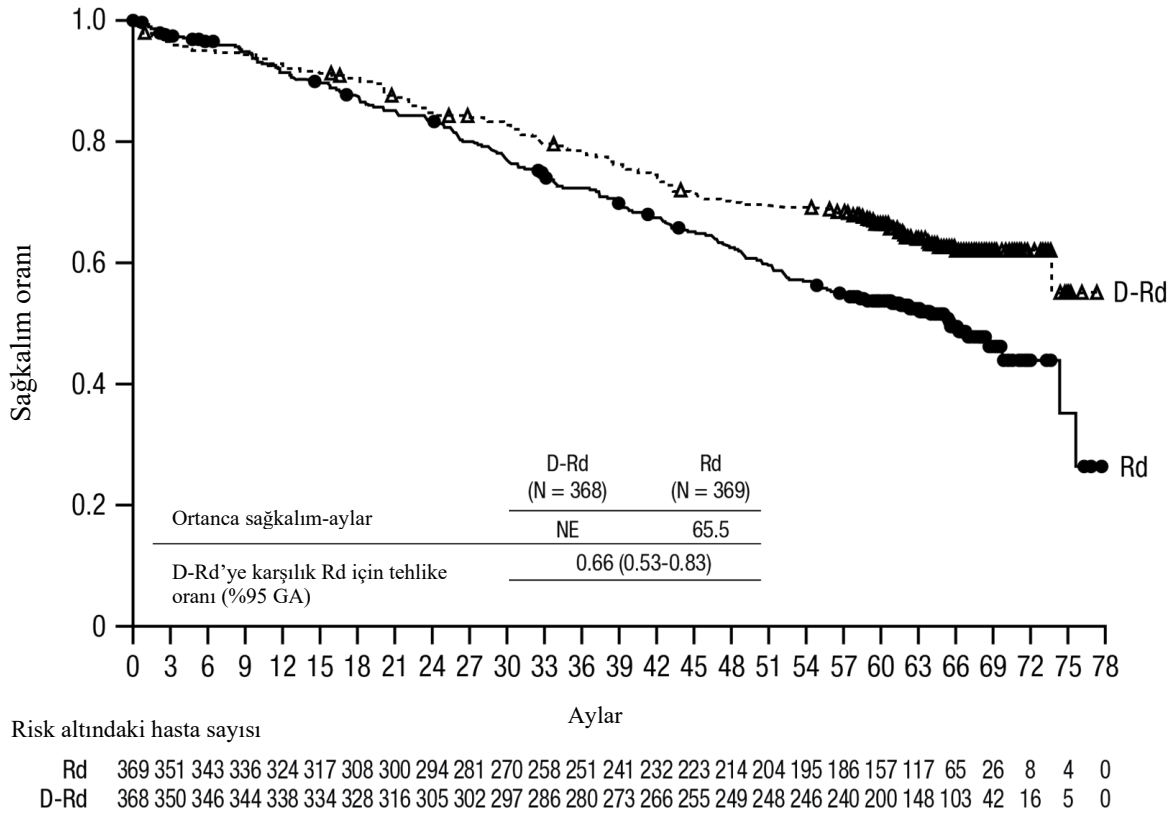
Şekil 2: MMY3008 çalışmasında Kaplan-Meier OS eğrisi
